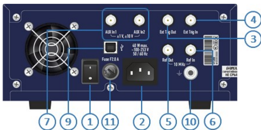
Рисунок – Задняя панель C1209
