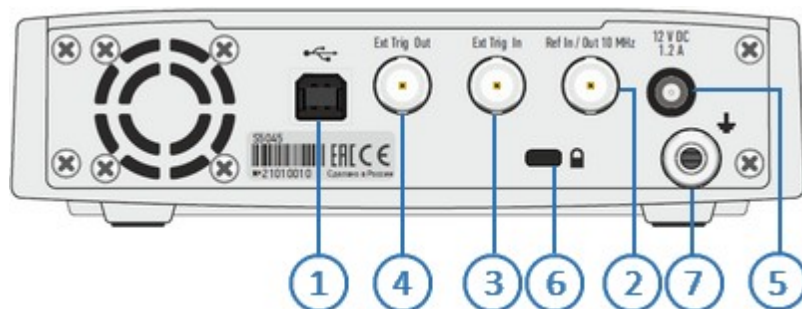
Рисунок – Задняя панель S5045, S5065, S5085
