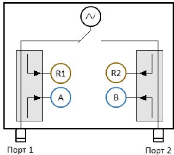
Рисунок — Структурная схема анализатора
