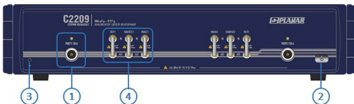
Рисунок – Передняя панель C2209
