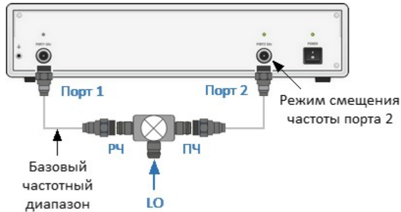
Рисунок – Измерение смесителя с использованием смещения частоты
