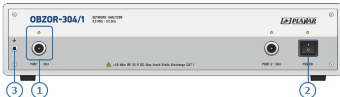
Рисунок – Передняя панель ОБЗОР-304/1
