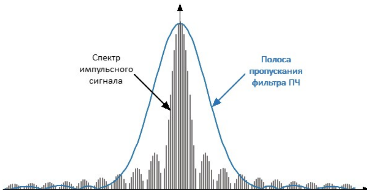
Рисунок – Широкополосное детектирование
