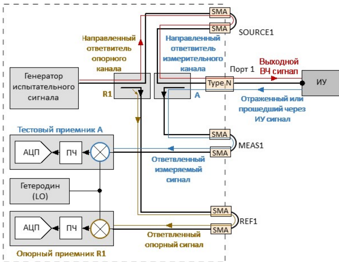
Рисунок – Анализатор C2209, распространение сигнала в общем режиме
