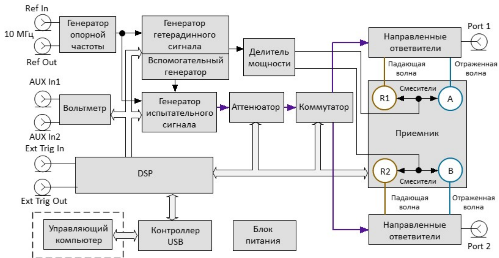
Рисунок – Структурная схема анализаторов
