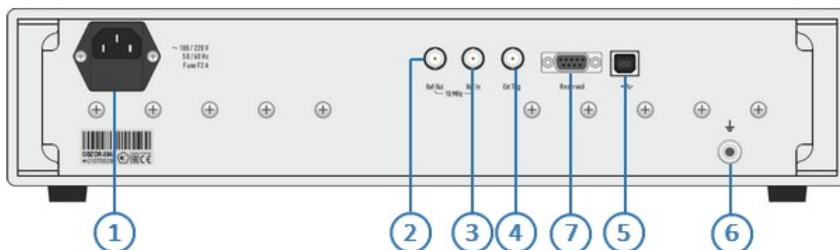
Рисунок – Задняя панель ОБЗОР-304/1
