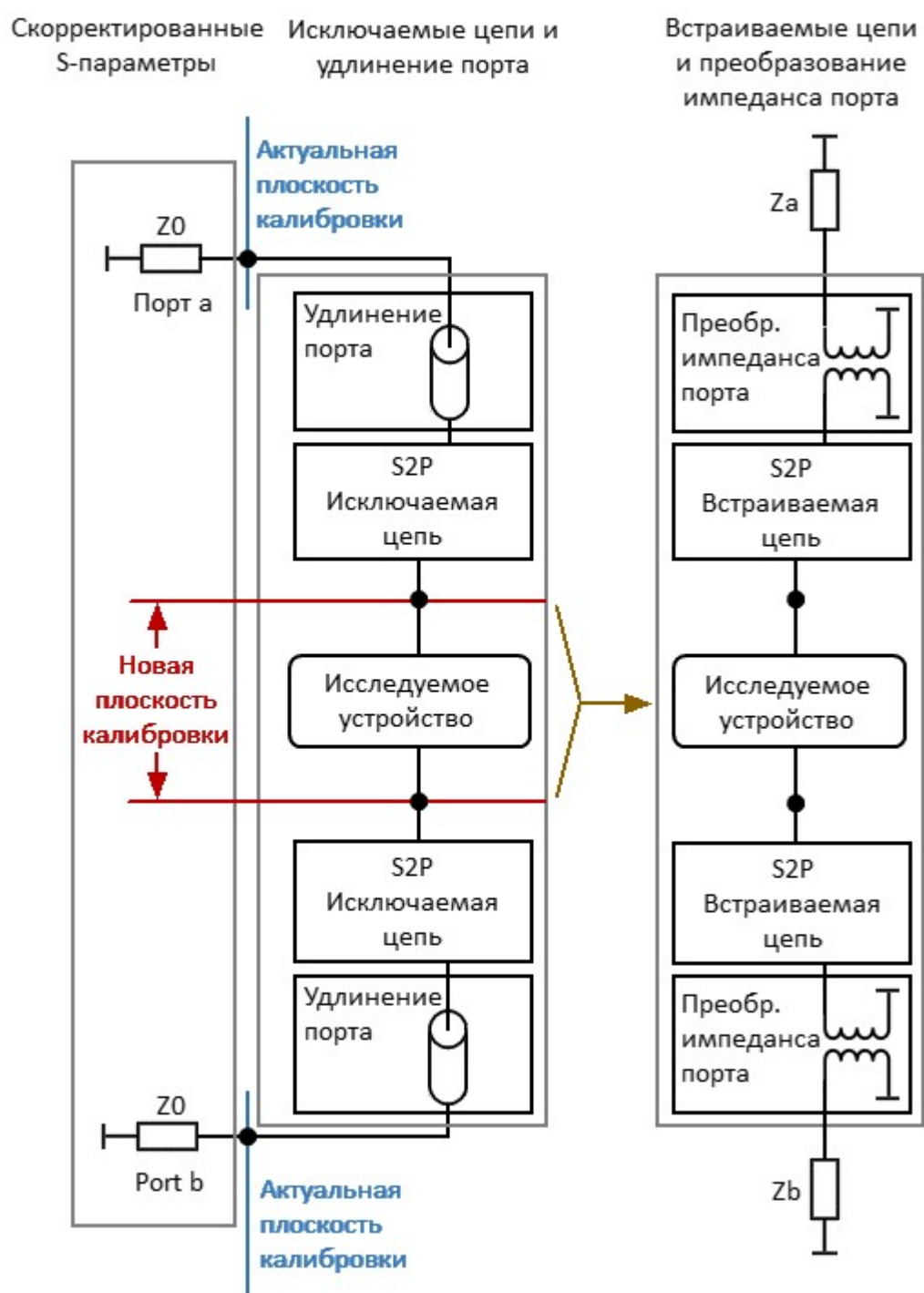
Рисунок – Логическая схема функции моделирования оснастки
