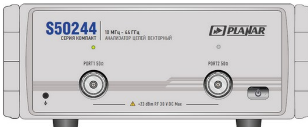
Рисунок – Передняя панель S50244
