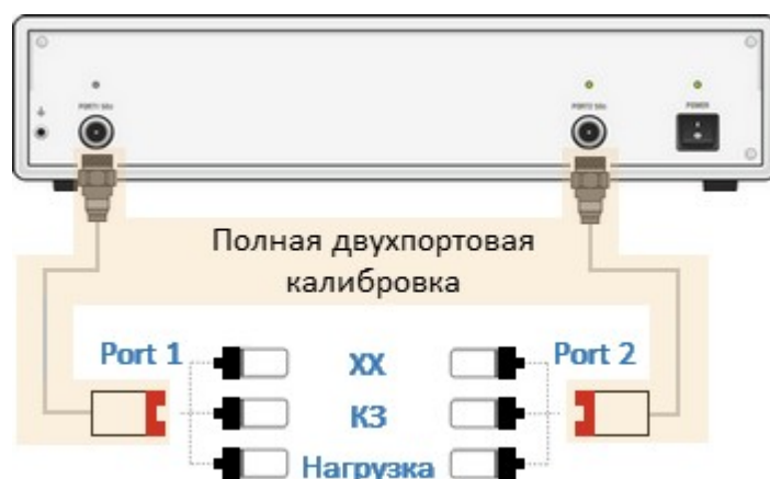
Рисунок – Первый этап калибровки с неизвестной перемычкой SOLR
