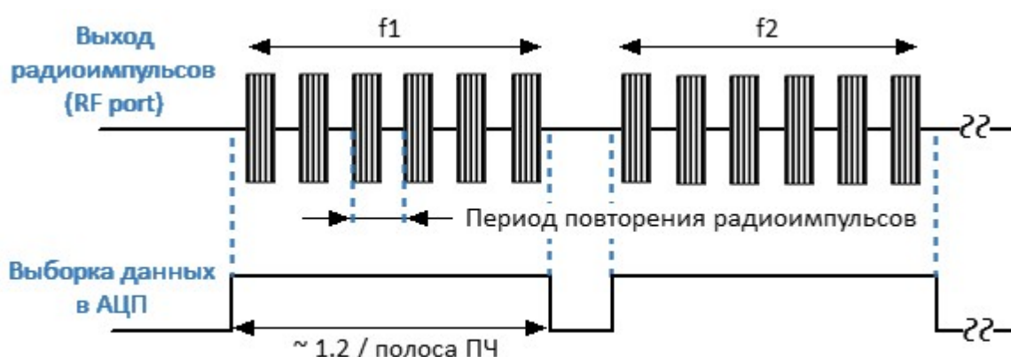
Рисунок – Асинхронный импульсный режим
