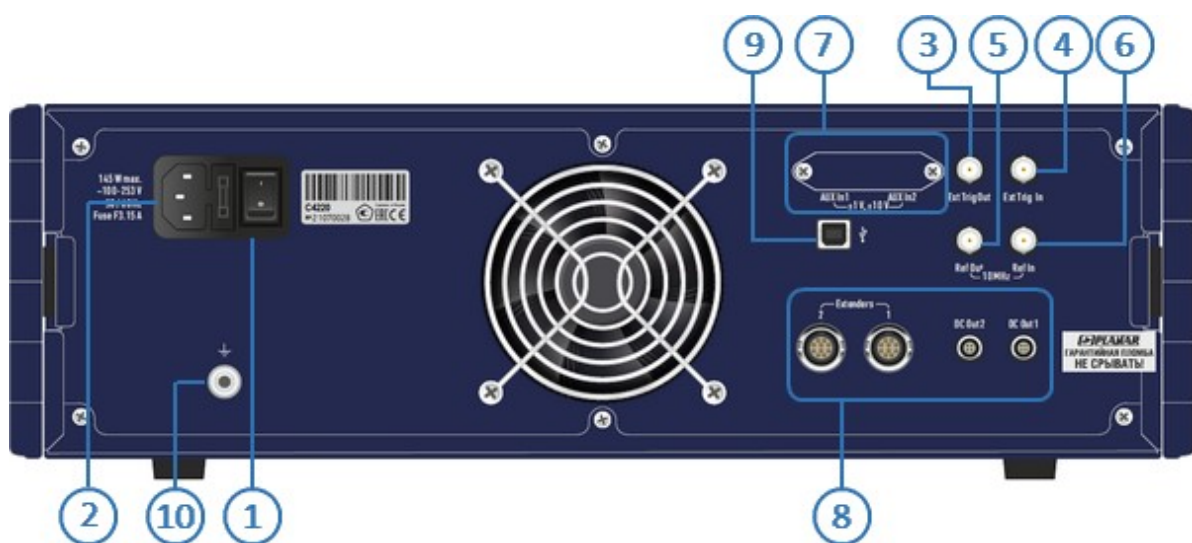
Рисунок – Задняя панель C4220
