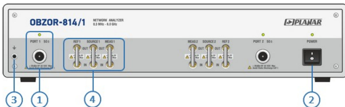
Рисунок – Передняя панель ОБЗОР-814/1
