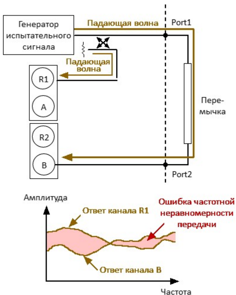
Рисунок – Ошибка частотной неравномерности передачи
