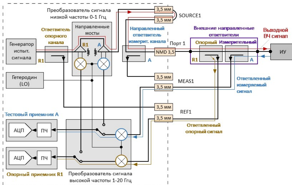
Рисунок – Анализатор C2220, распространение сигнала в режиме прямого доступа
