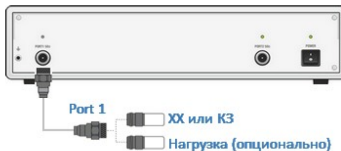
Рисунок – Калибровка нормализации отражения
