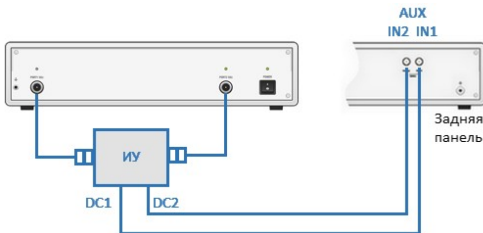
Рисунок – Пример схемы подключения ИУ к вольтметру
