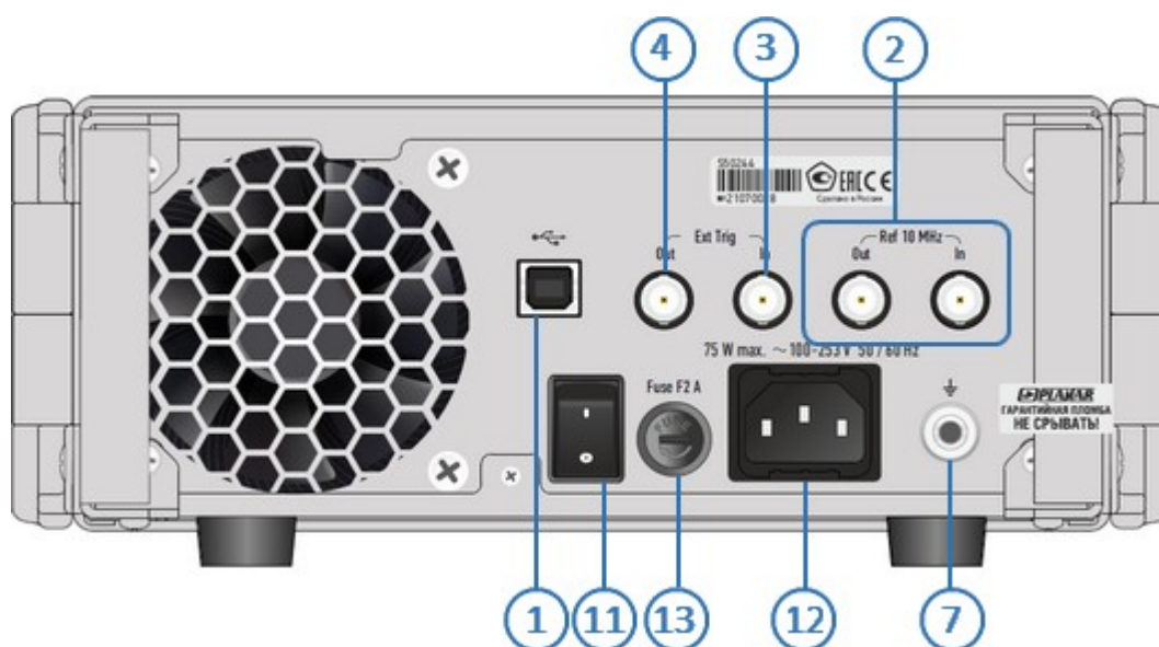
Рисунок – Задняя панель S50244
