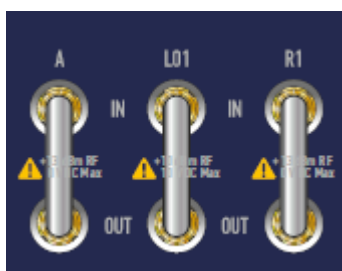
Рисунок – Расположение дополнительных разъемов анализатора C4220
