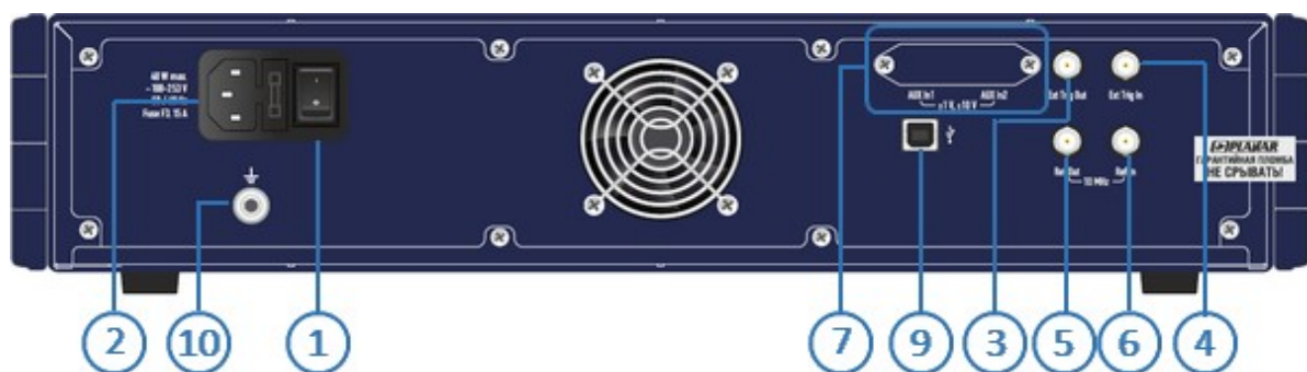
Рисунок – Задняя панель C2209
