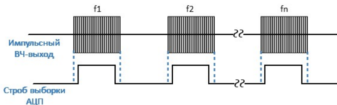
Рисунок – Метод «Точка в импульсе»
