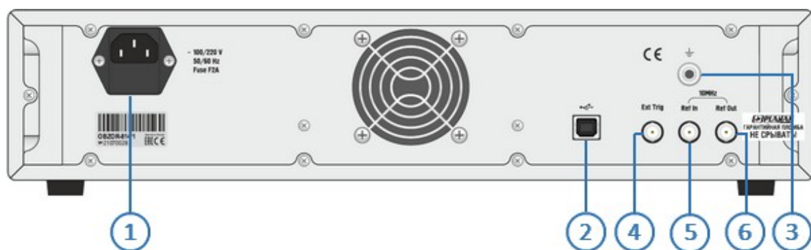
Рисунок – Задняя панель ОБЗОР-804/1 и ОБЗОР-814/1
