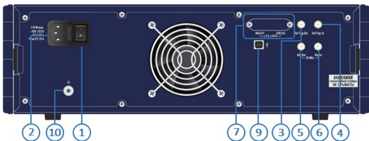
Рисунок – Задняя панель C1220, C2220
