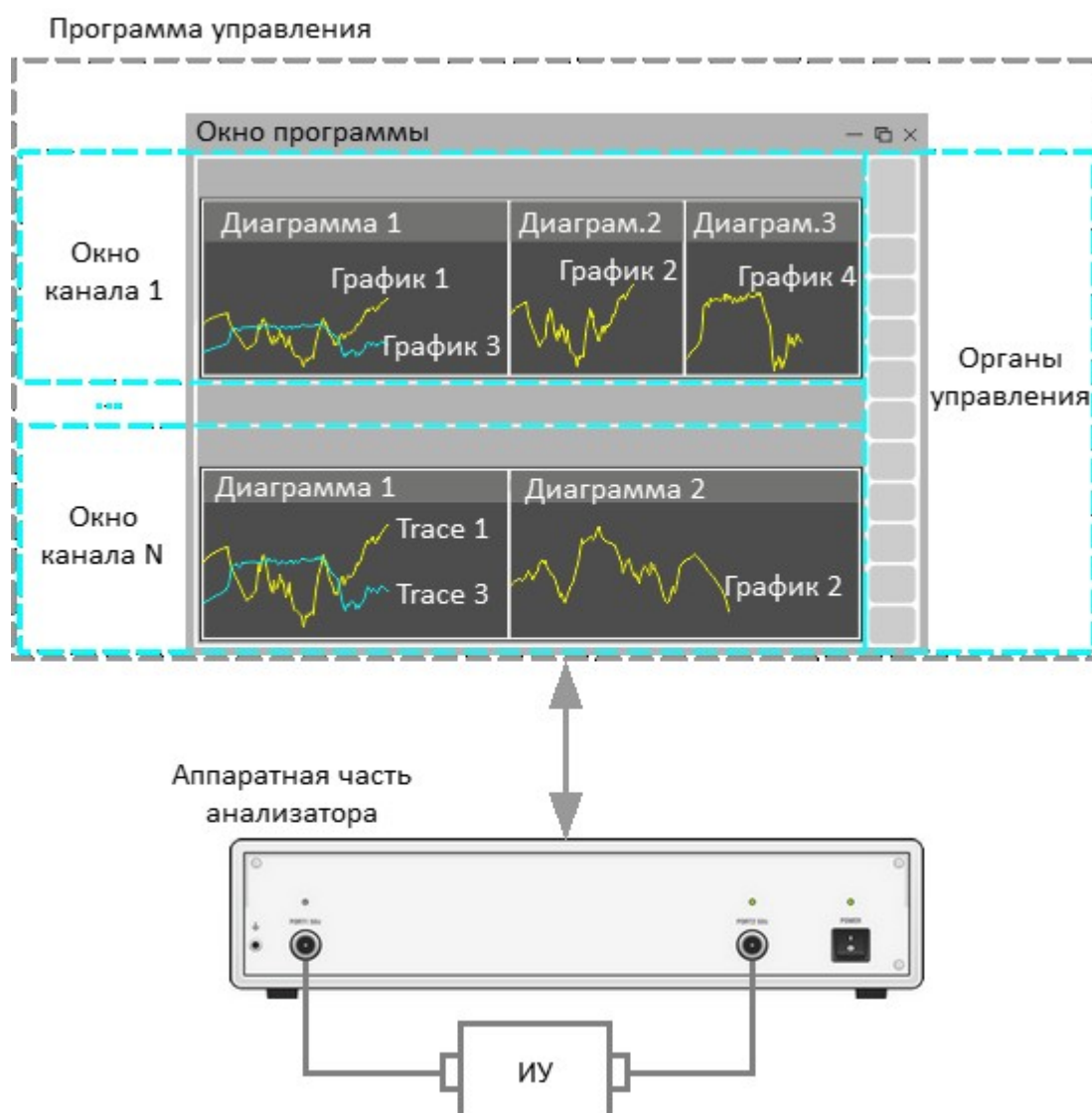
Рисунок – Иерархия средств измерения, обработки и отображения информации
