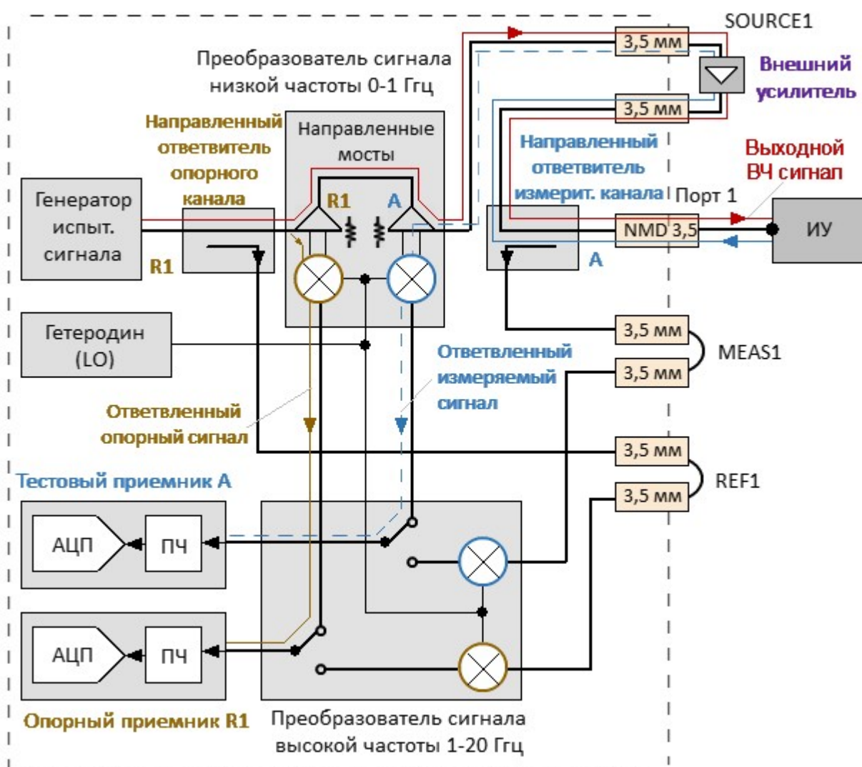
Рисунок – Анализатор C2220, распространение сигнала с внешним усилителем в тракте генератора (диапазон от 100 кГц до 1 ГГц)
