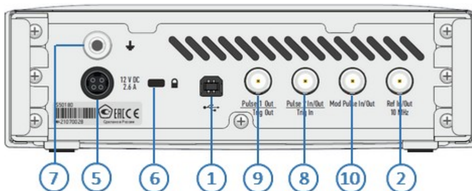
Рисунок – Задняя панель S50180
