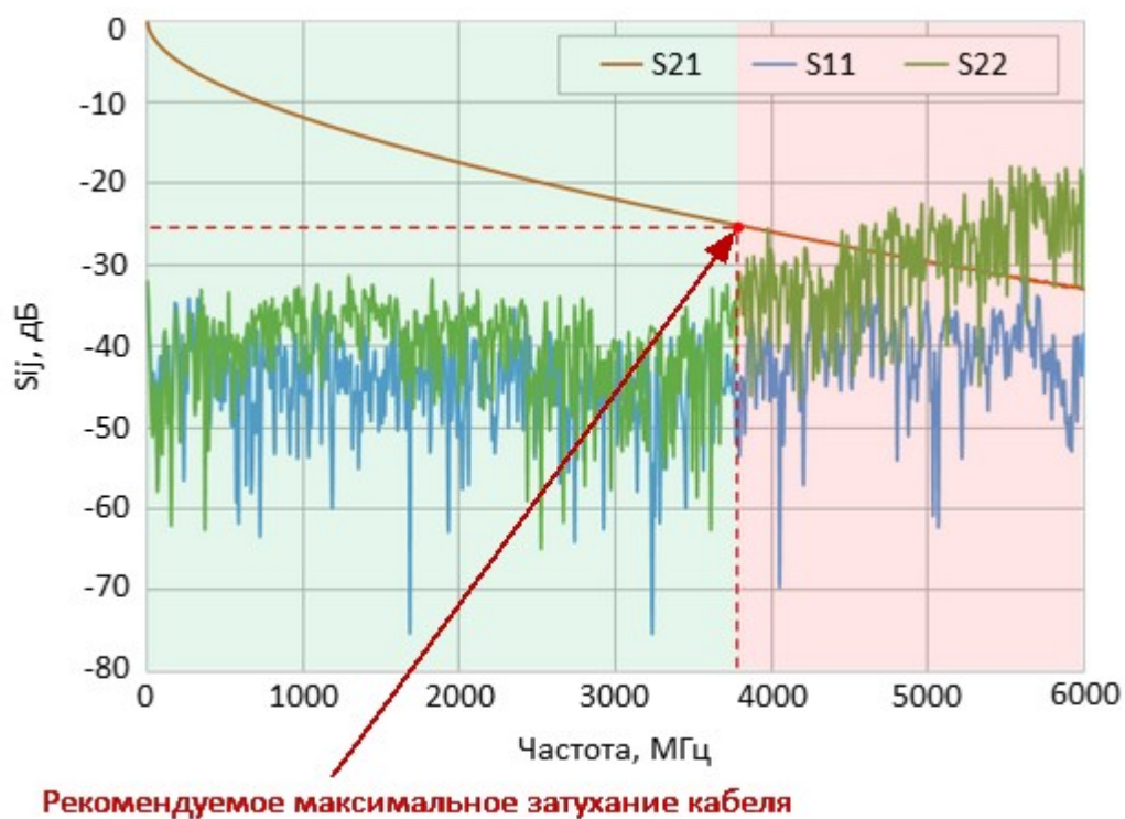
Рисунок – Коэффициенты передачи и отражения S_{11}^{ACMB} , S_{21}^{ACMB} , S_{22}^{ACMB}
