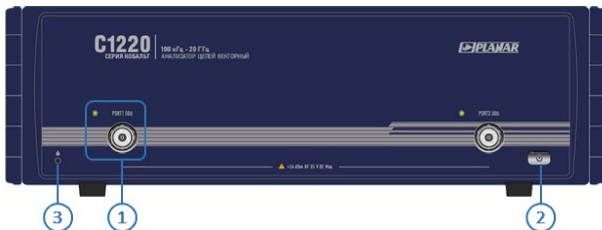
Рисунок – Передняя панель C1220
