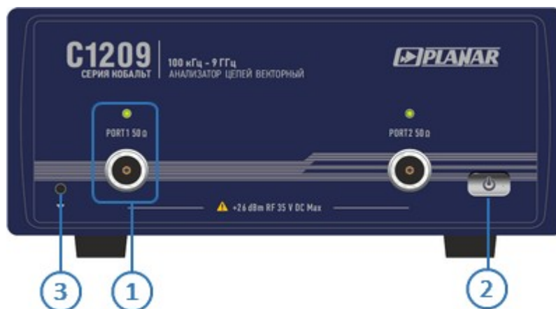
Рисунок – Передняя панель C1209
