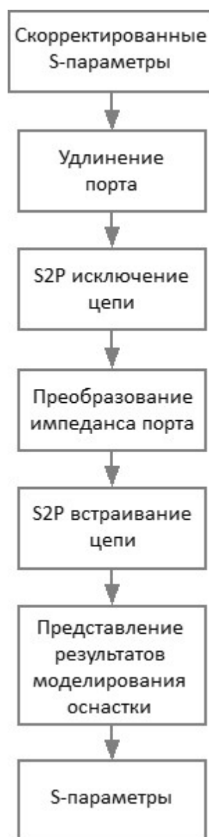
Рисунок – Блок-схема обработки данных при моделировании оснастки
