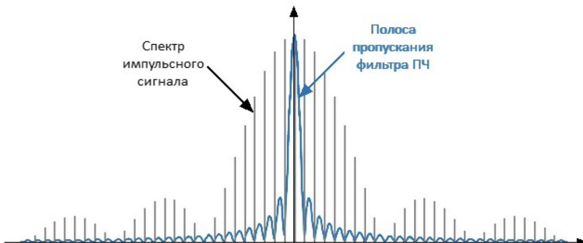
Рисунок – Узкополосное детектирование
