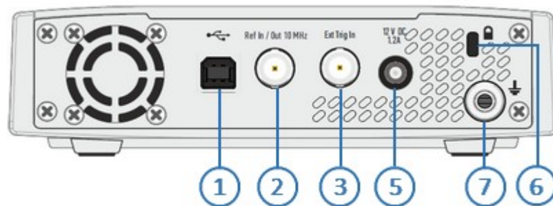
Рисунок – Задняя панель S5075, S5048
