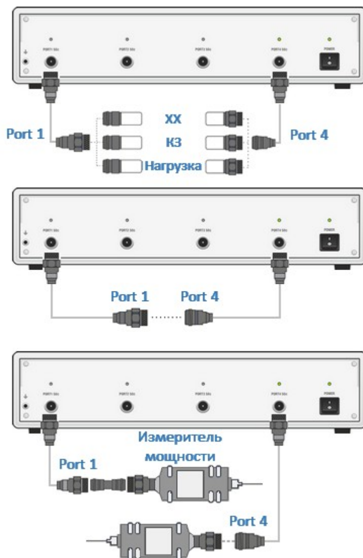
Рисунок – Схема скалярной калибровки смесителей
