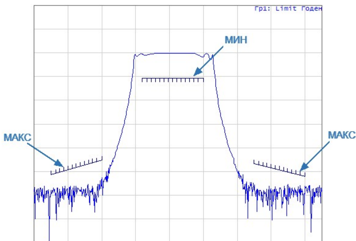
Рисунок – Пример линии пределов
