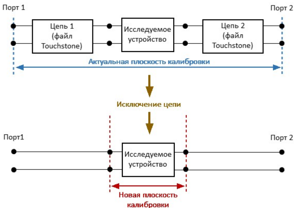
Рисунок – Исключение цепи
