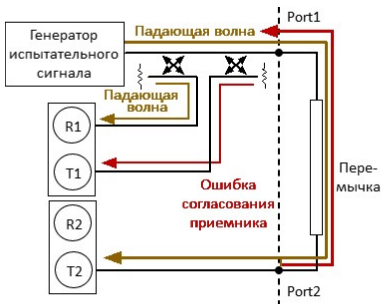
Рисунок – Ошибка согласования приемника
