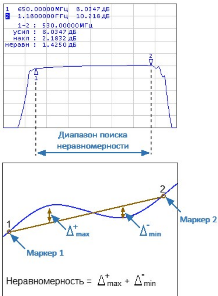
Рисунок – Поиск неравномерности
