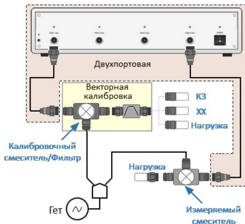
Рисунок – Векторная калибровка смесителей
