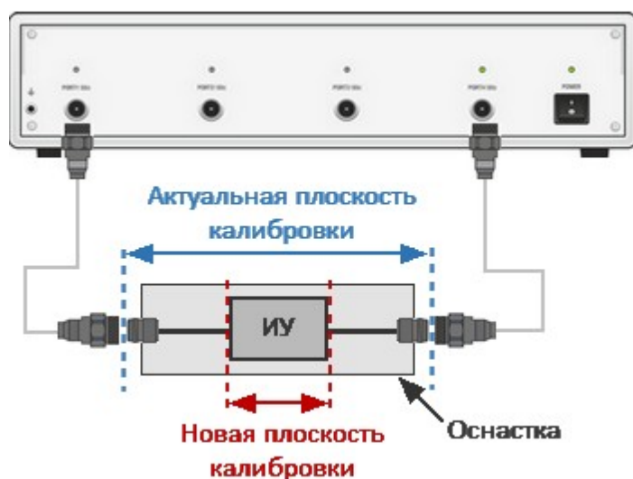
Рисунок – Удлинение портов
