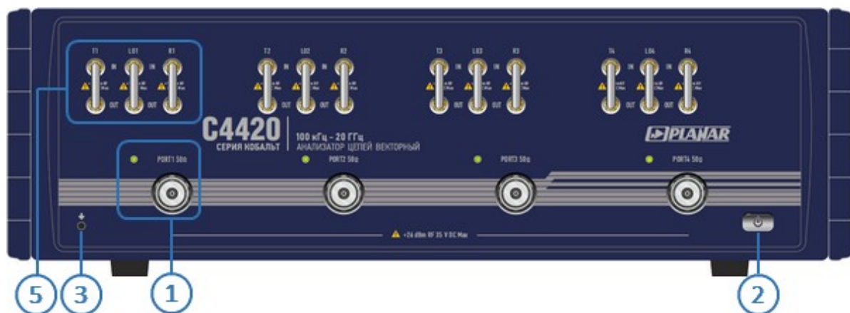
Рисунок – Передняя панель C4420
