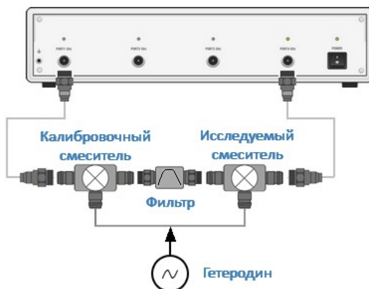
Рисунок – Схема векторного измерения смесителя
