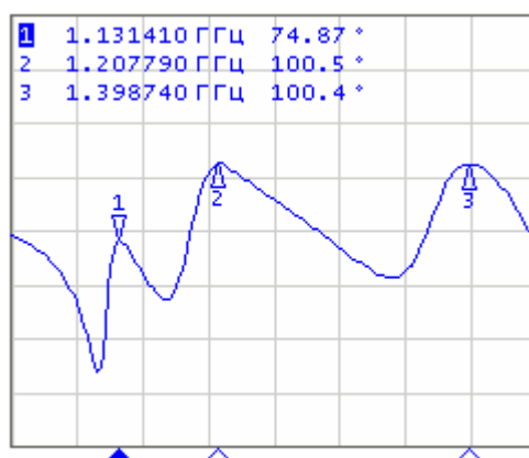
Рисунок – Пример положительных пиков
