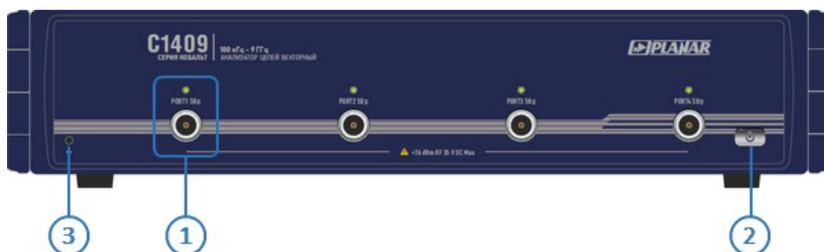
Рисунок – Передняя панель C1409
