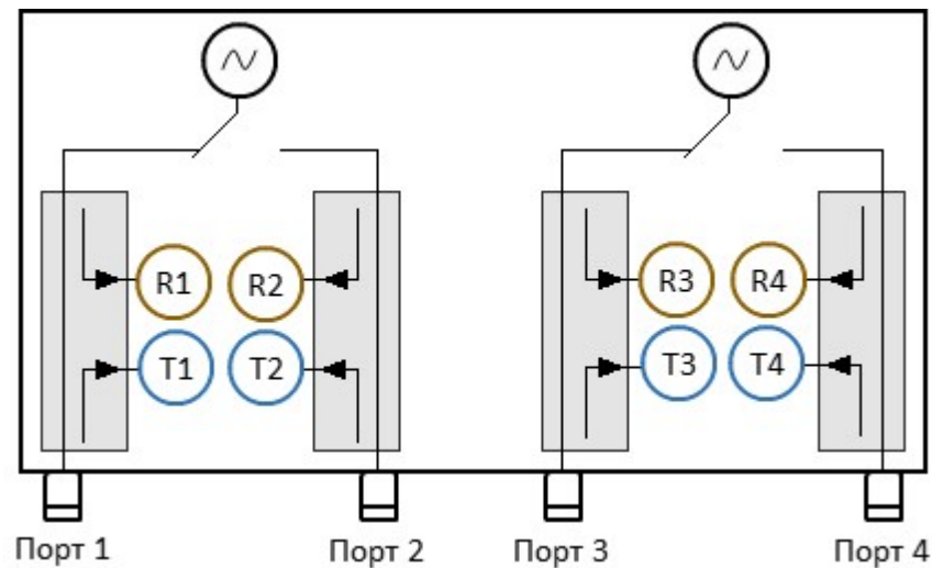
Рисунок — Структурная схема анализатора
