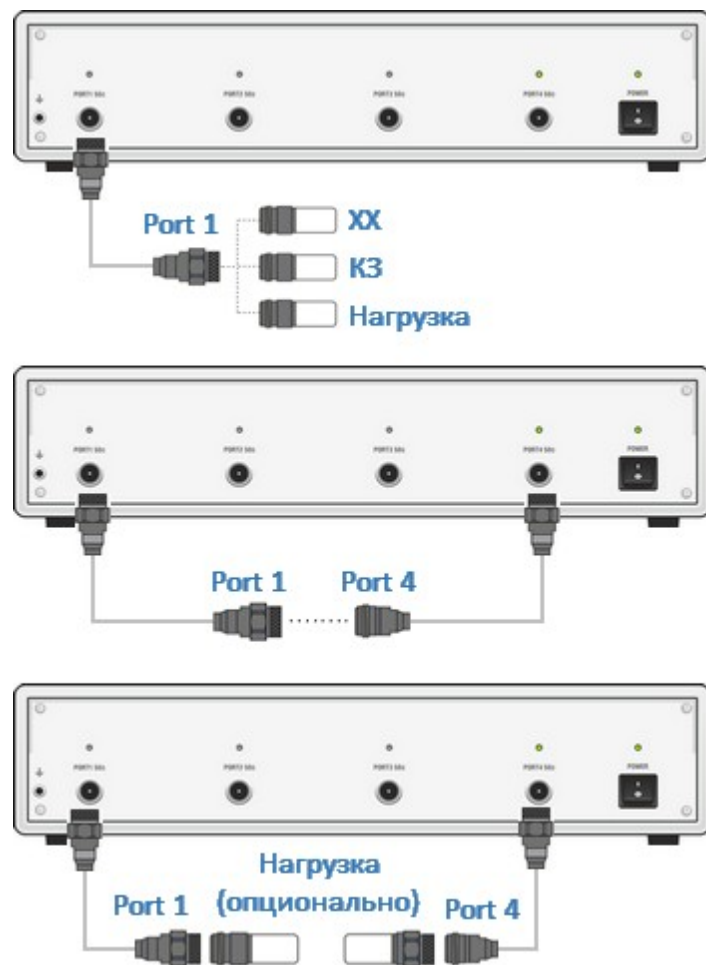
Рисунок – Однонаправленная двухпортовая калибровка
