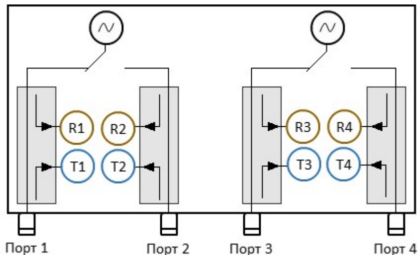
Рисунок – Структурная схема четырехпортового анализатора
