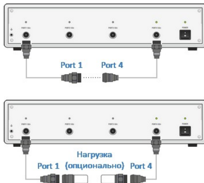
Рисунок – Калибровка нормализации передачи
