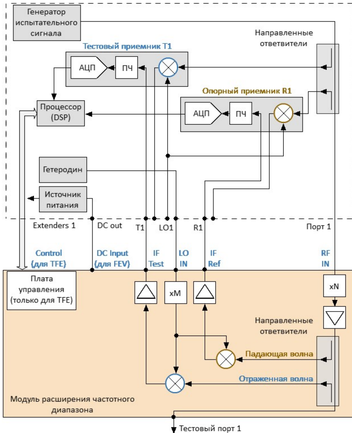
Рисунок – Структурная схема подключения модуля к анализатору
