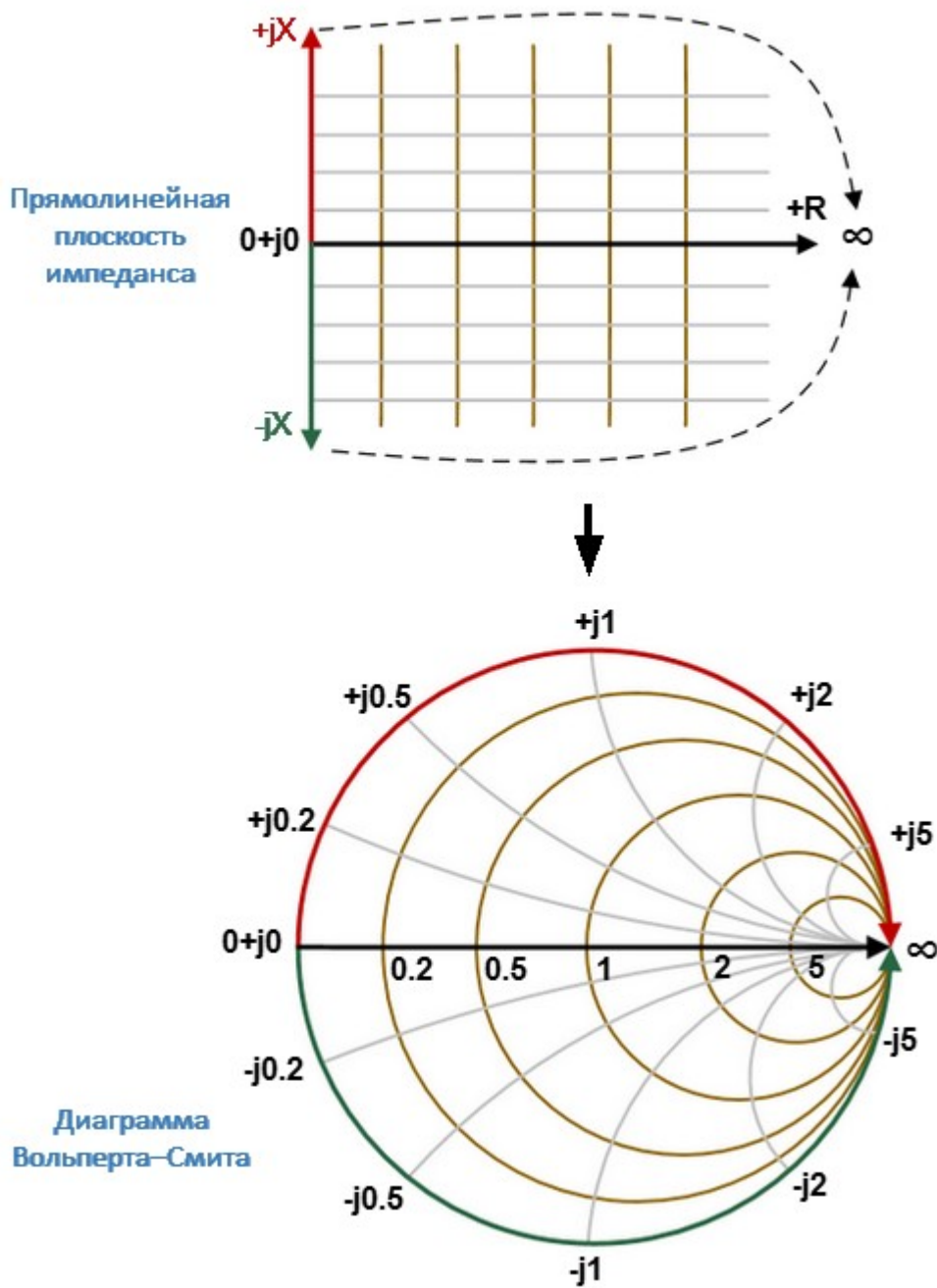
Рисунок — Преобразование прямолинейной плоскости импеданса в диаграмму Вольперта-Смита
