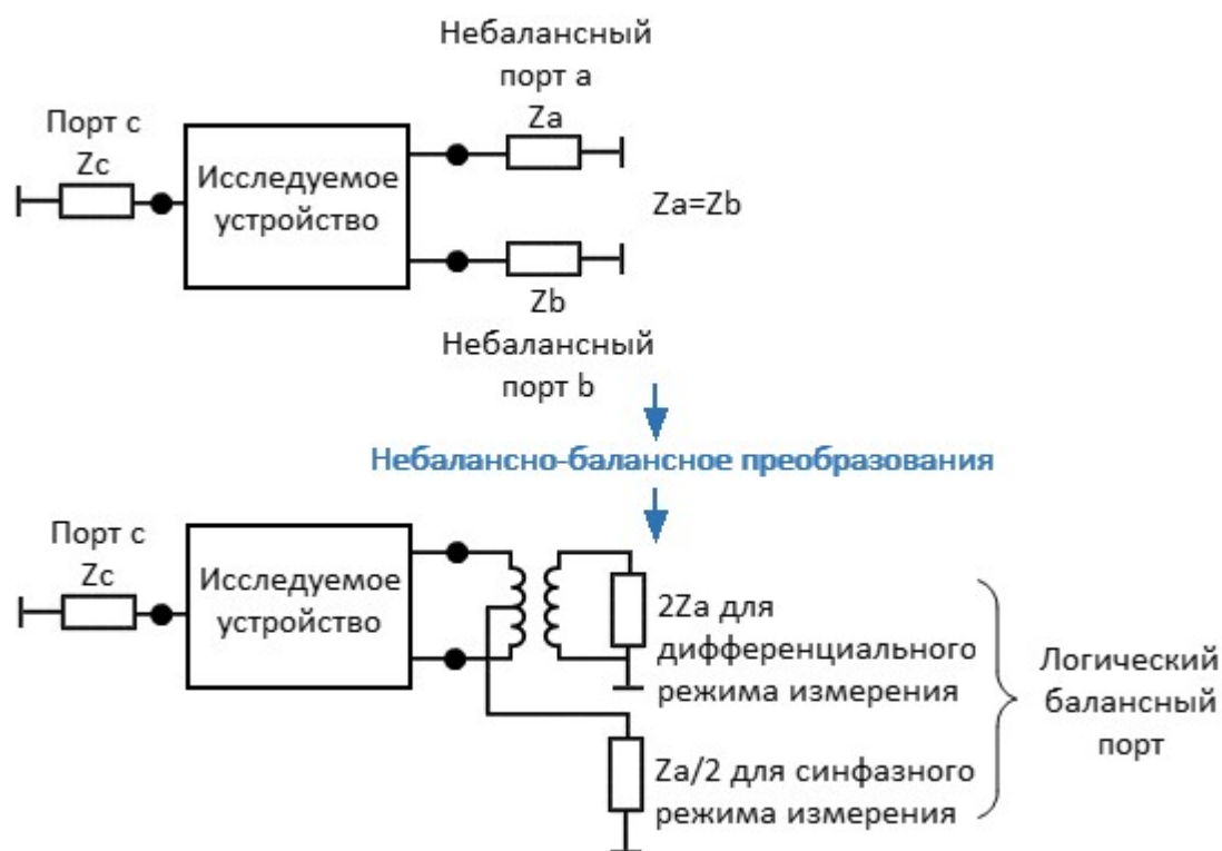
Рисунок – Схема небалансно-балансного преобразования
