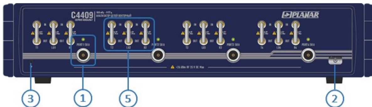
Рисунок – Передняя панель C4409
