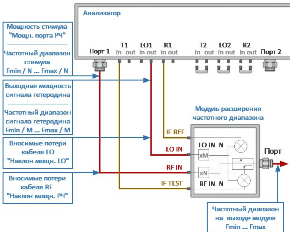
Рисунок – Схема установки параметров модуля
