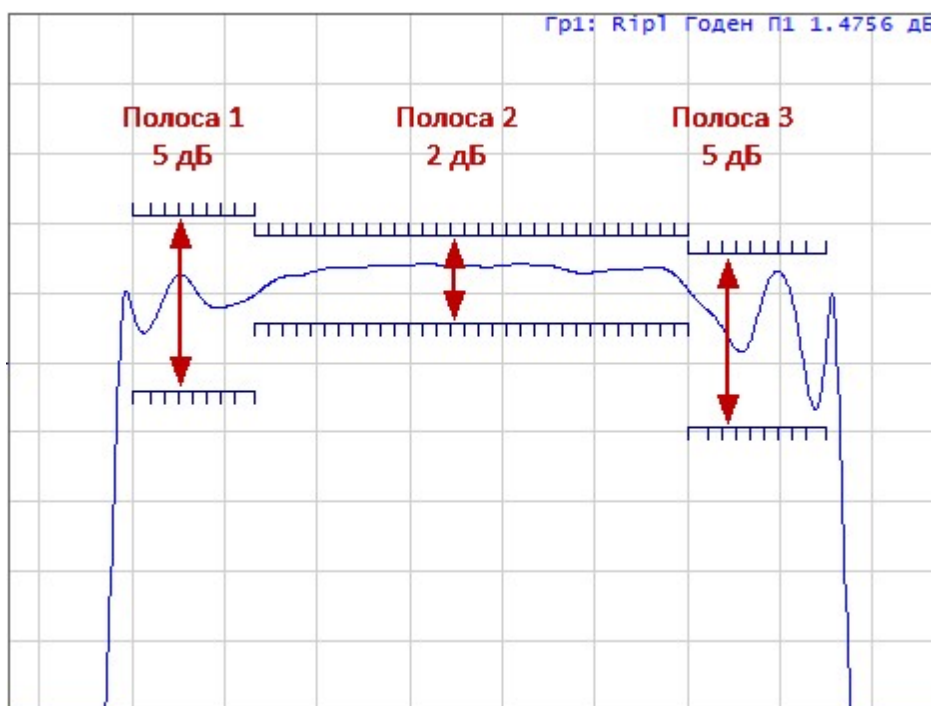
Рисунок – Пример пределов пульсаций
