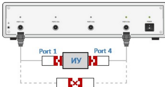
Рисунок – Пример устройства с не присоединяемыми портами (соединители одного типа)
