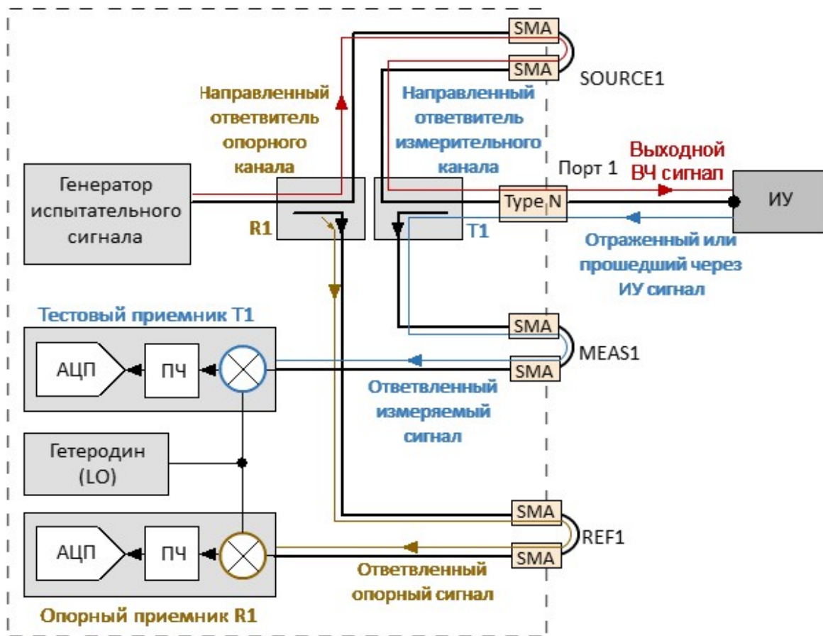
Рисунок – Анализатор C2409, распространение сигнала в общем режиме
