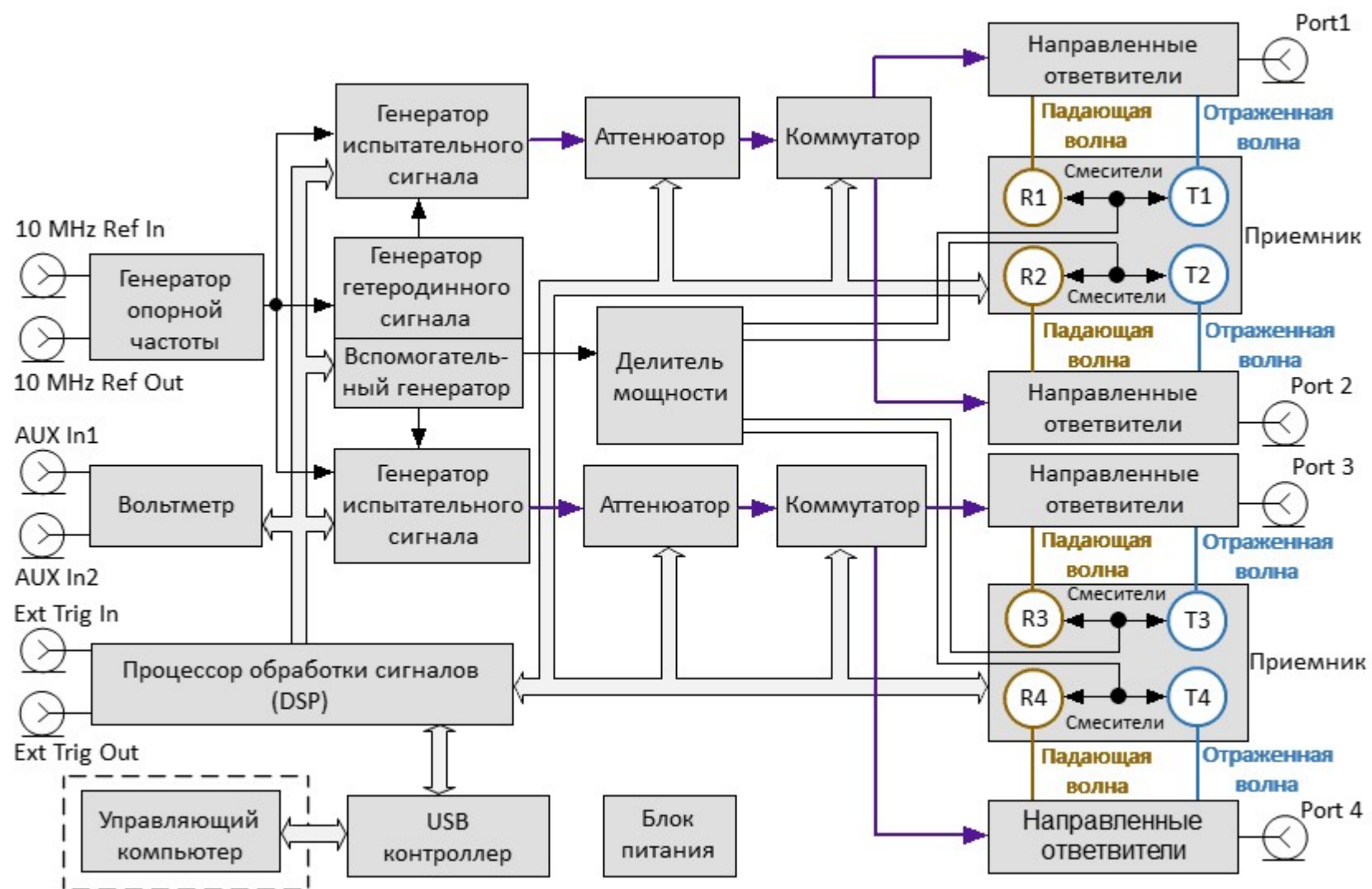
Рисунок – Структурная схема анализаторов
