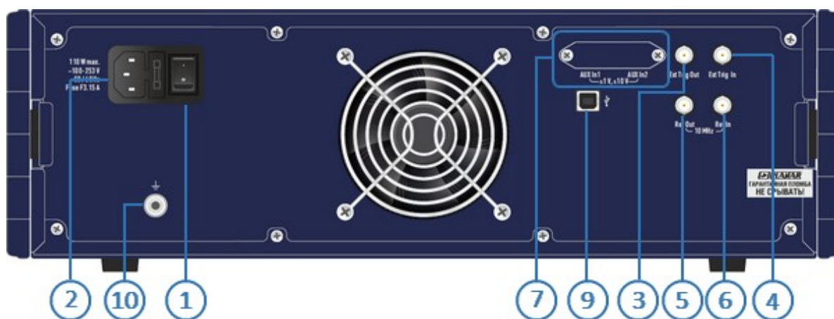
Рисунок – Задняя панель S1420, S2420
