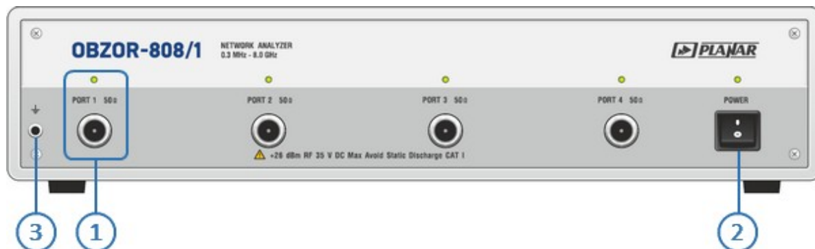
Рисунок – Передняя панель ОБЗОР-808/1
