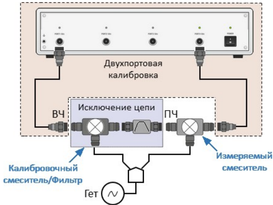
Рисунок – Векторные измерения смесителей
