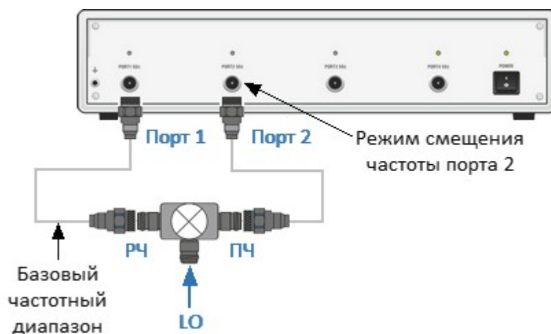
Рисунок – Измерение смесителя с использованием смещения частоты
