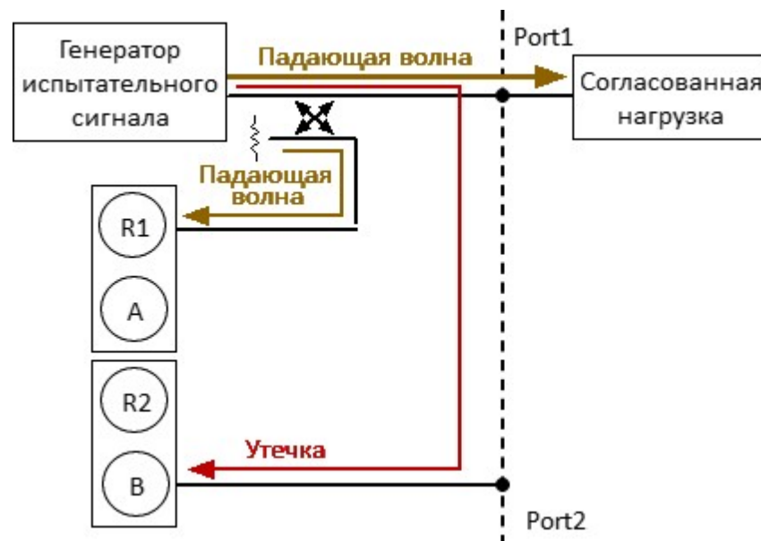
Рисунок – Ошибка развязки
