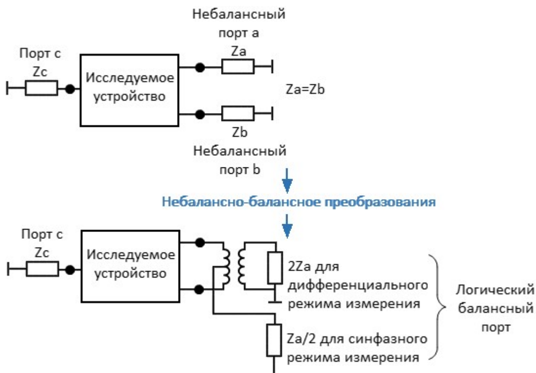
Рисунок – Схема небалансно-балансного преобразования
