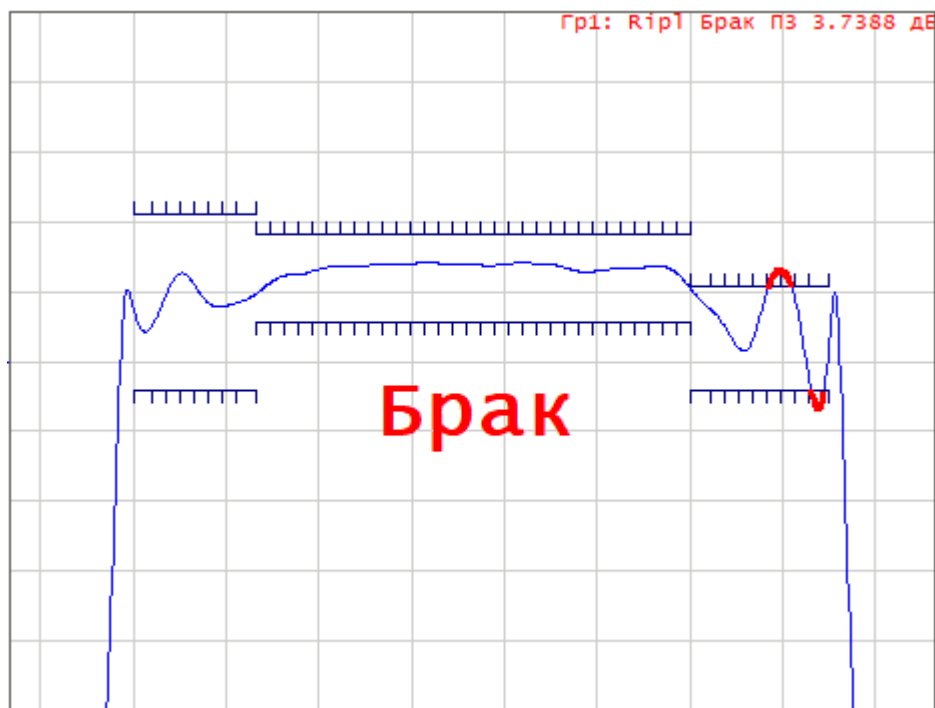
Рисунок – Пример отрицательных результатов испытания
