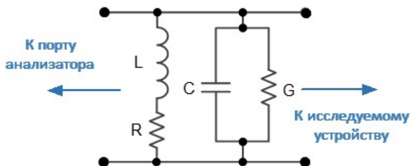
Рисунок – Предустановленная согласующая цепь
