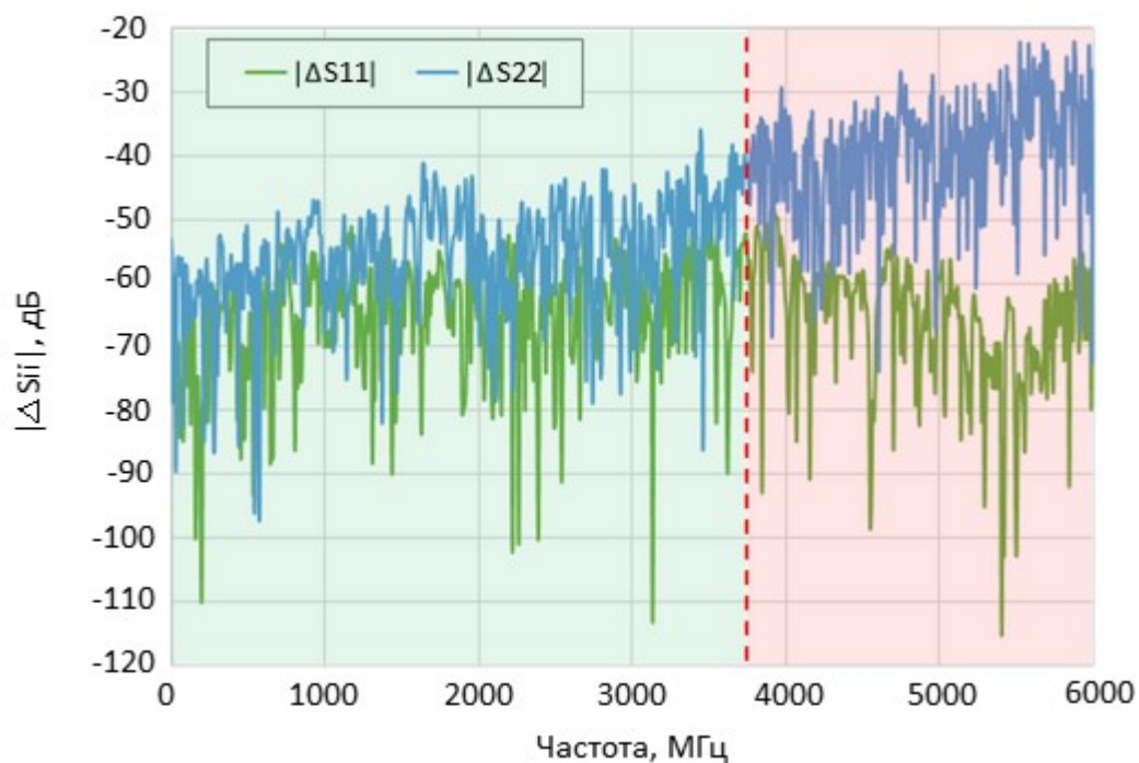
Рисунок – Отклонение коэффициента отражения \Delta|S_{ii}| = 20 \lg |S_{ii}^{ACMB} - S_{ii}^{BAЦ}|
