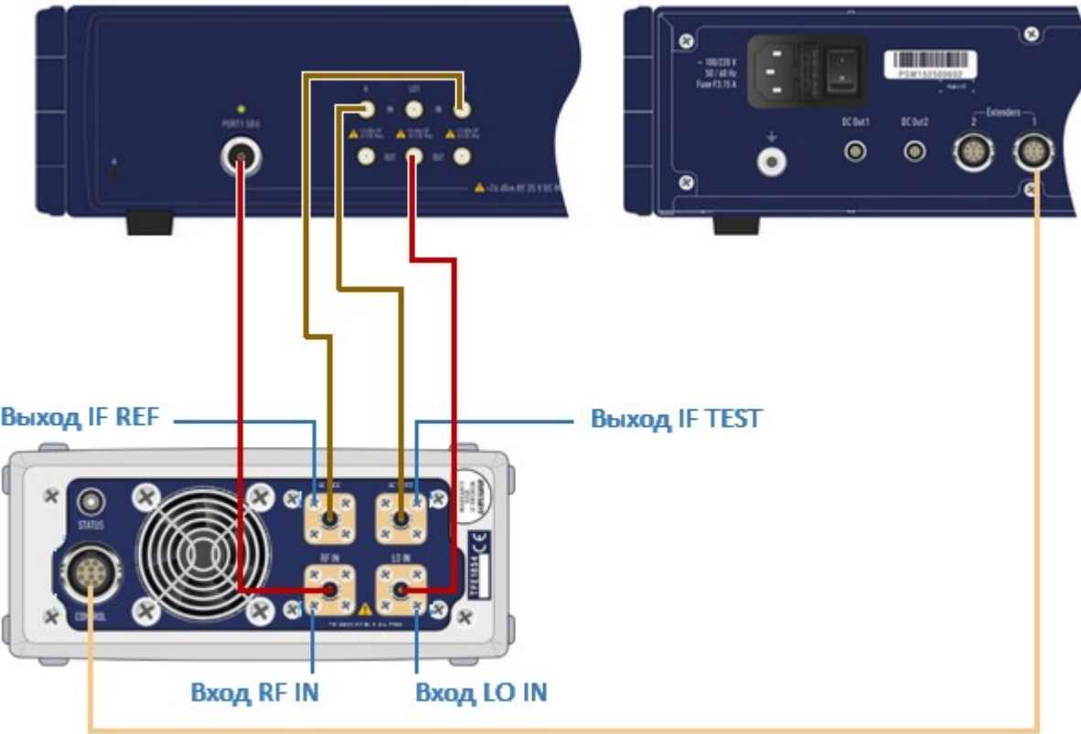
Рисунок – Схема подключения модуля TFE-1854 к анализатору
