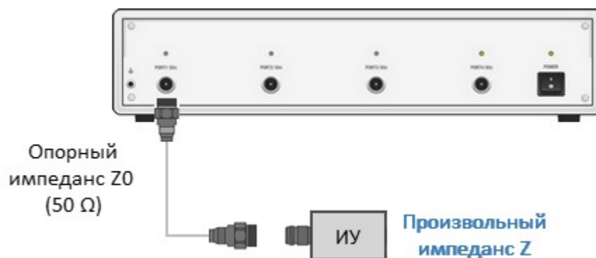
Рисунок – Пример измерения анализатором с опорным импедансом 50 Ом ИУ с произвольным импедансом
