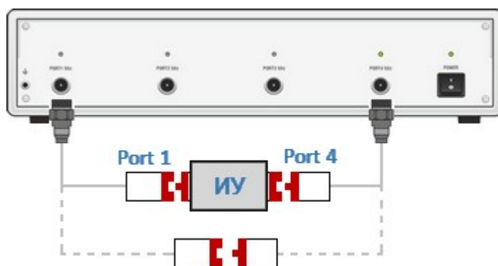
Рисунок – Пример устройства с присоединяемыми портами
