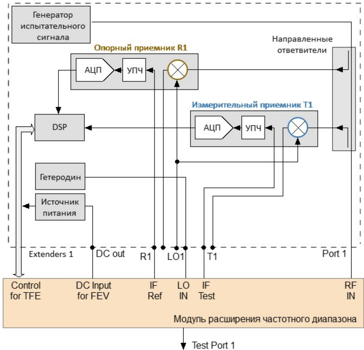
Рисунок – Подключение модуля расширения частотного диапазона
