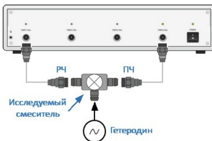
Рисунок – Схема скалярного измерения смесителя
