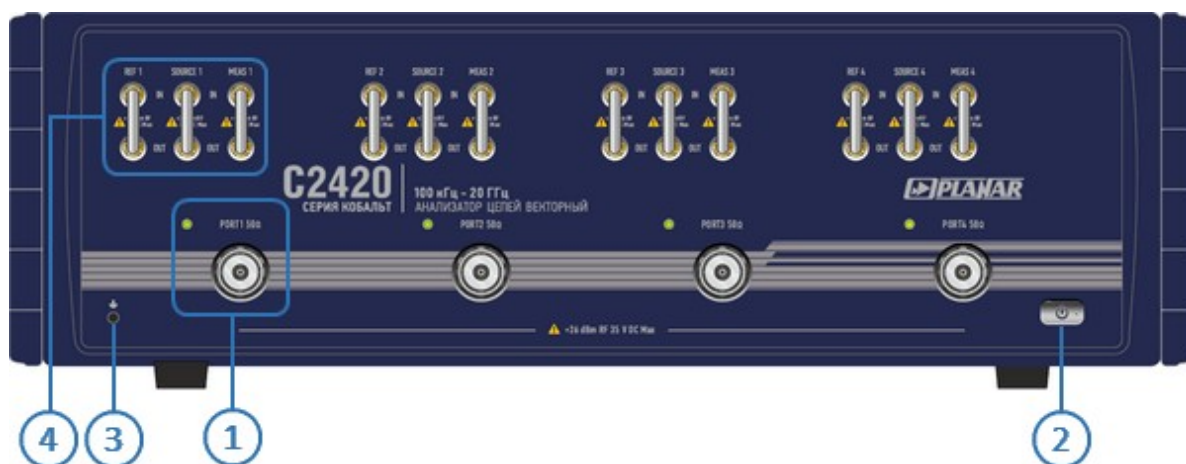
Рисунок – Передняя панель C2420
