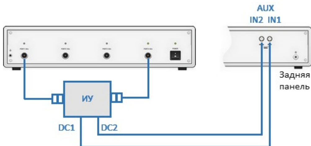
Рисунок – Пример схемы подключения ИУ к вольтметру
