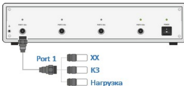
Рисунок – Полная однопортовая калибровка
