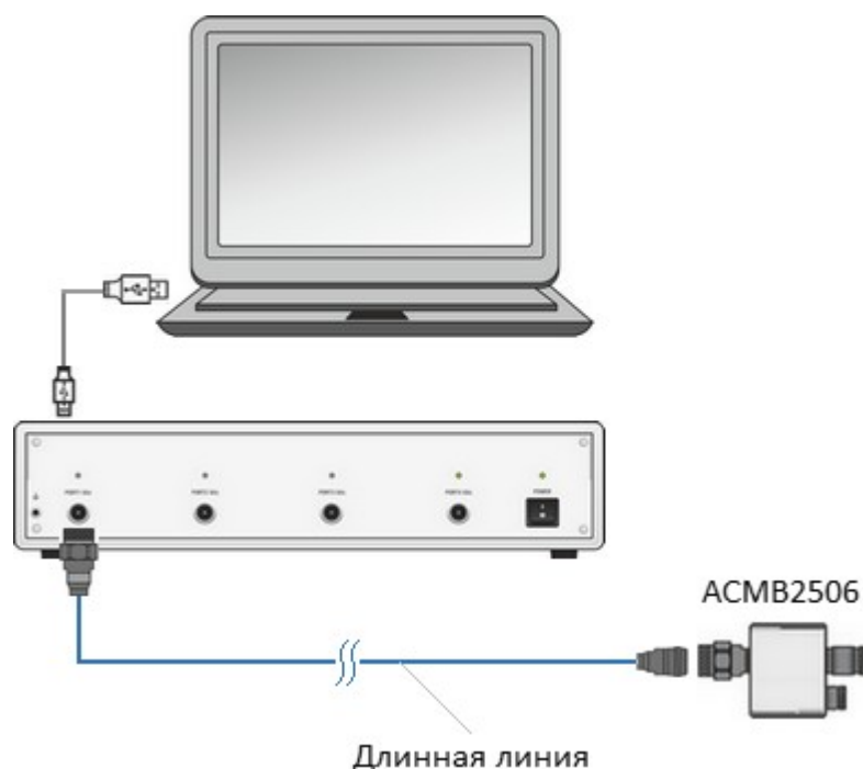
Рисунок – Подключение ACMB2506 в режиме измерения длинной линии
