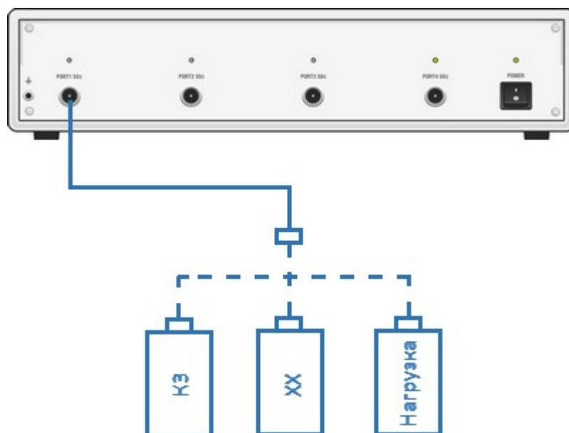
Рисунок – Схема полной однопортовой калибровки
