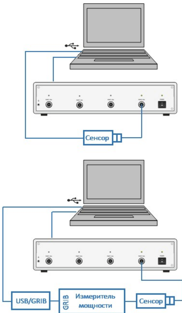
Рисунок – Пример подключения измерителя мощности
