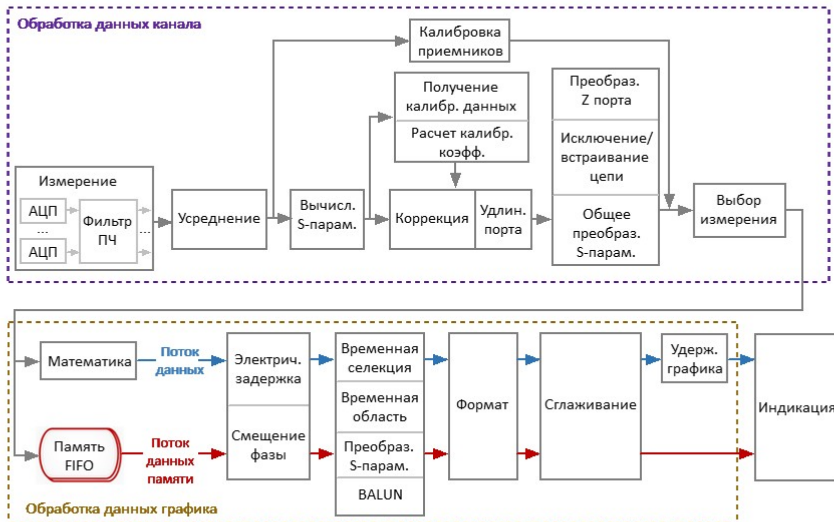
Рисунок – Блок-схема конвейера обработки данных
