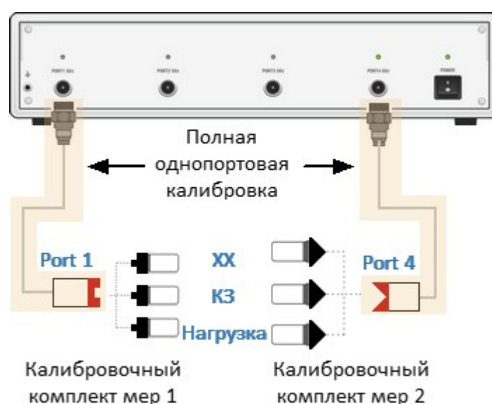
Рисунок – Однопортовая калибровка перед добавлением неизвестной перемычки
