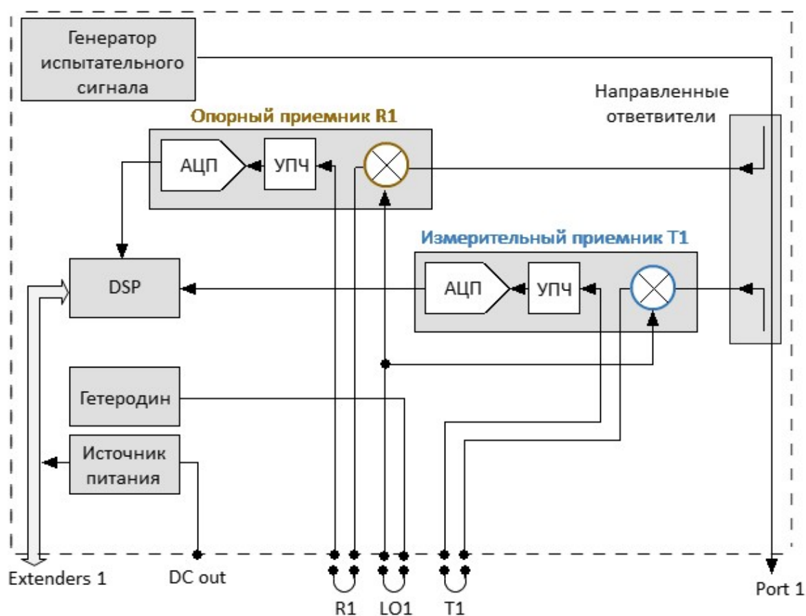
Рисунок – Анализатор с возможностью расширения диапазона частот
