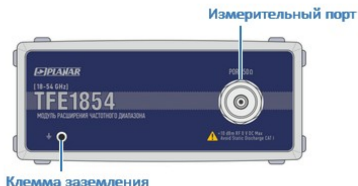
Рисунок – Передняя панель TFE-1854
