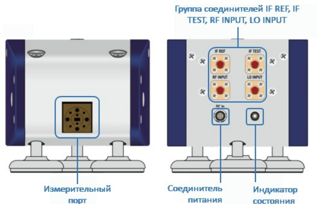
Рисунок – Передняя и задняя панели модуля FEV
