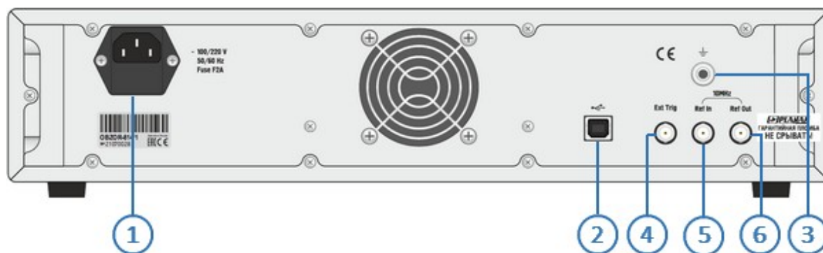
Рисунок - Задняя панель ОБЗОР-808/1
