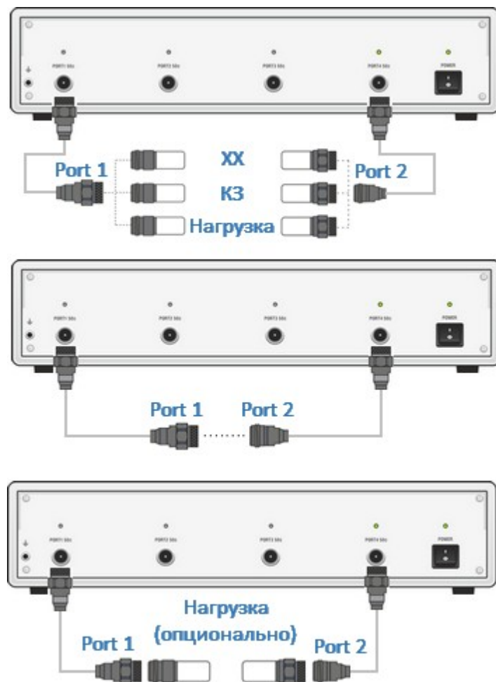
Рисунок – Полная двухпортовая калибровка
