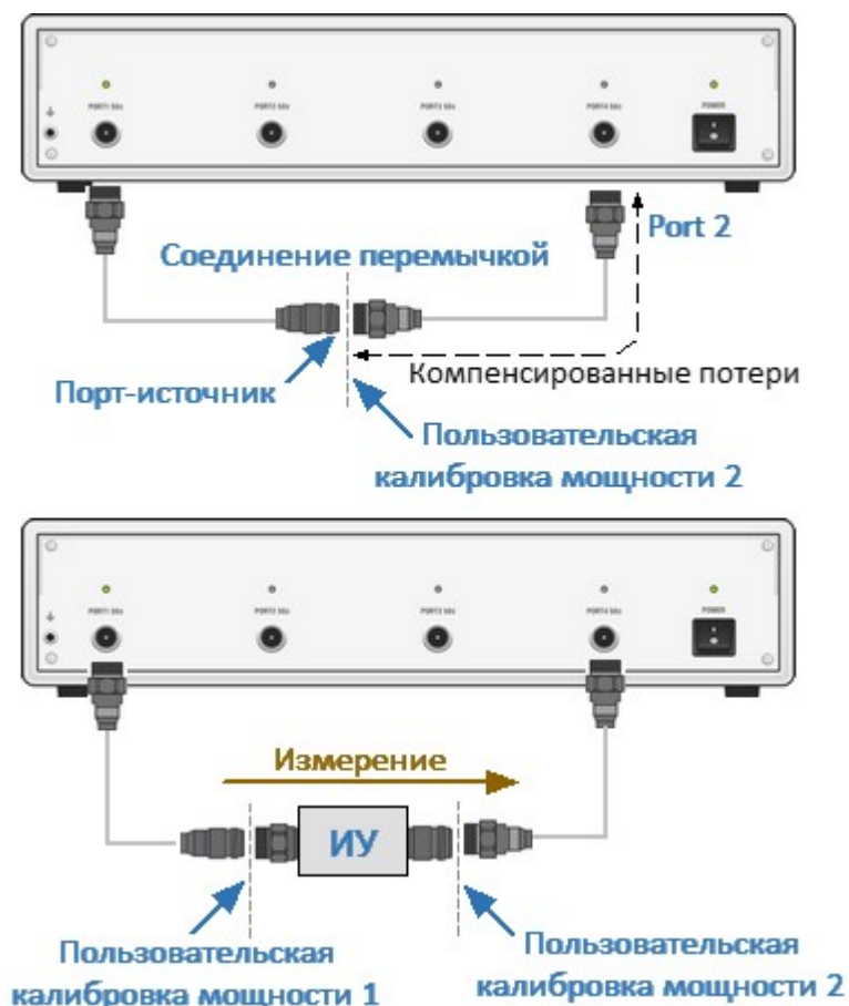
Рисунок – Калибровка приемников
