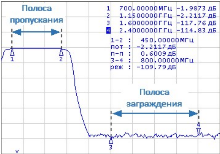
Рисунок – Характеристики полосового фильтра
