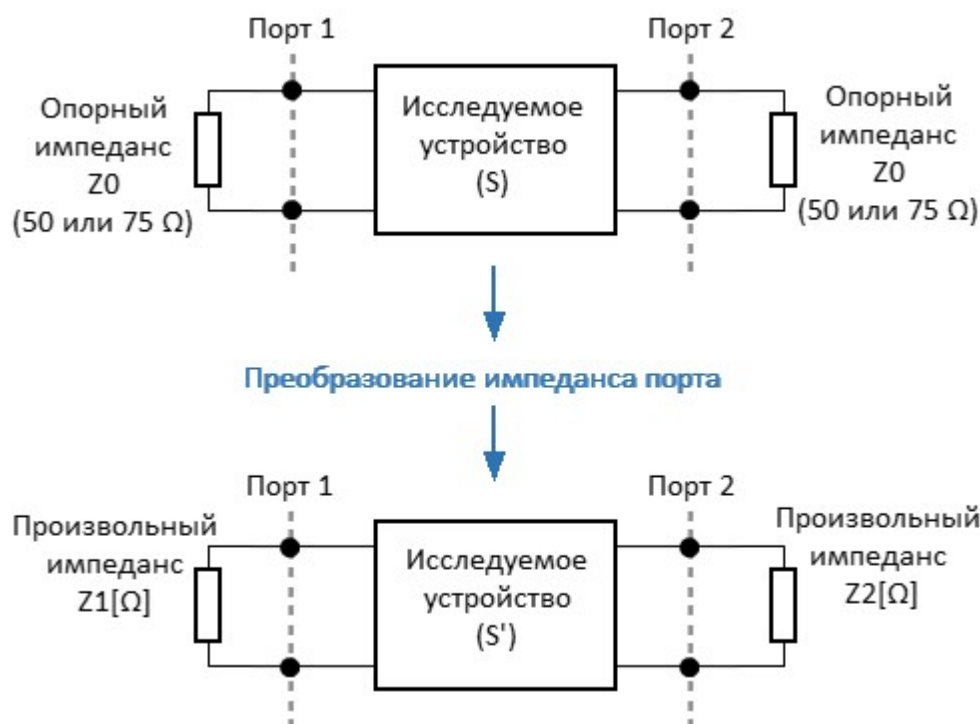
Рисунок – Преобразование импеданса порта
