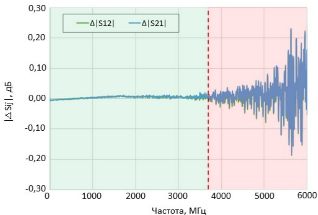
Рисунок – Отклонение коэффициента передачи \Delta|S_{ij}| = |S_{ij}^{ACMB} - S_{ij}^{BAЦ}|
