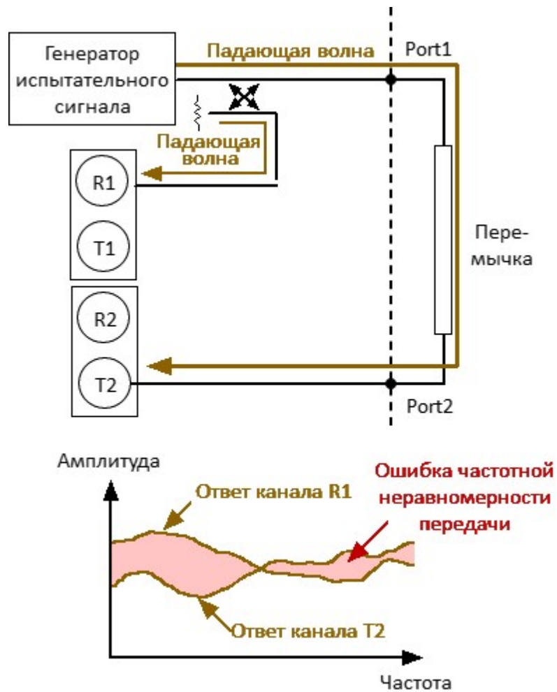
Рисунок – Ошибка частотной неравномерности передачи
