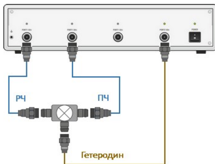
Рисунок – Свободный порт используется как источник сигнала гетеродина
