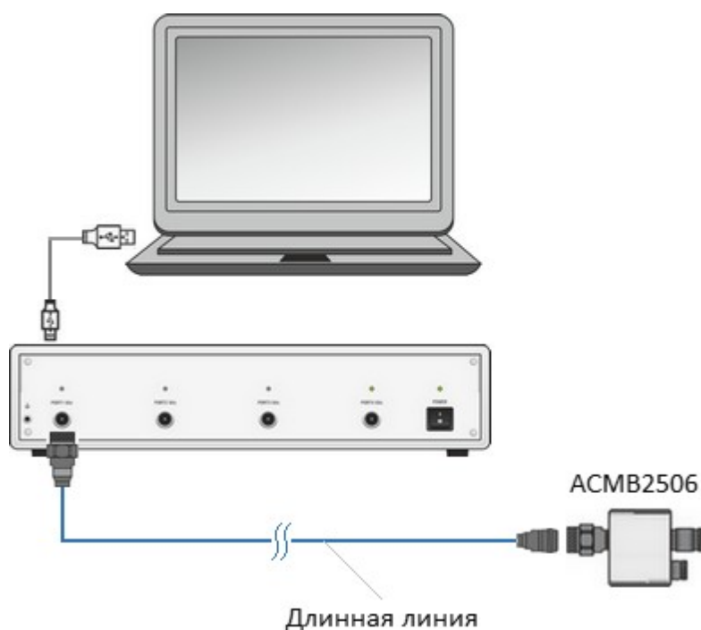
Рисунок – Схема измерения S-параметров длинной линии с помощью ACMB2506
