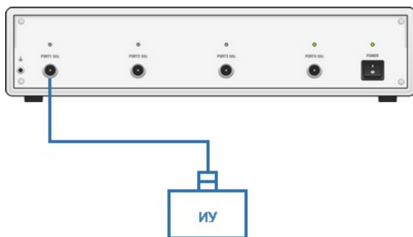
Рисунок – Схема измерения коэффициента отражения ИУ
