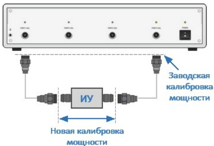
Рисунок – Калибровка мощности
