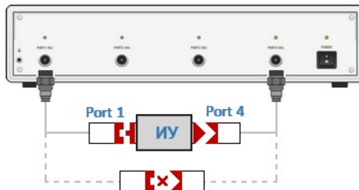
Рисунок – Пример устройства с не присоединяемыми портами (соединители имеют разный тип разъемов)
