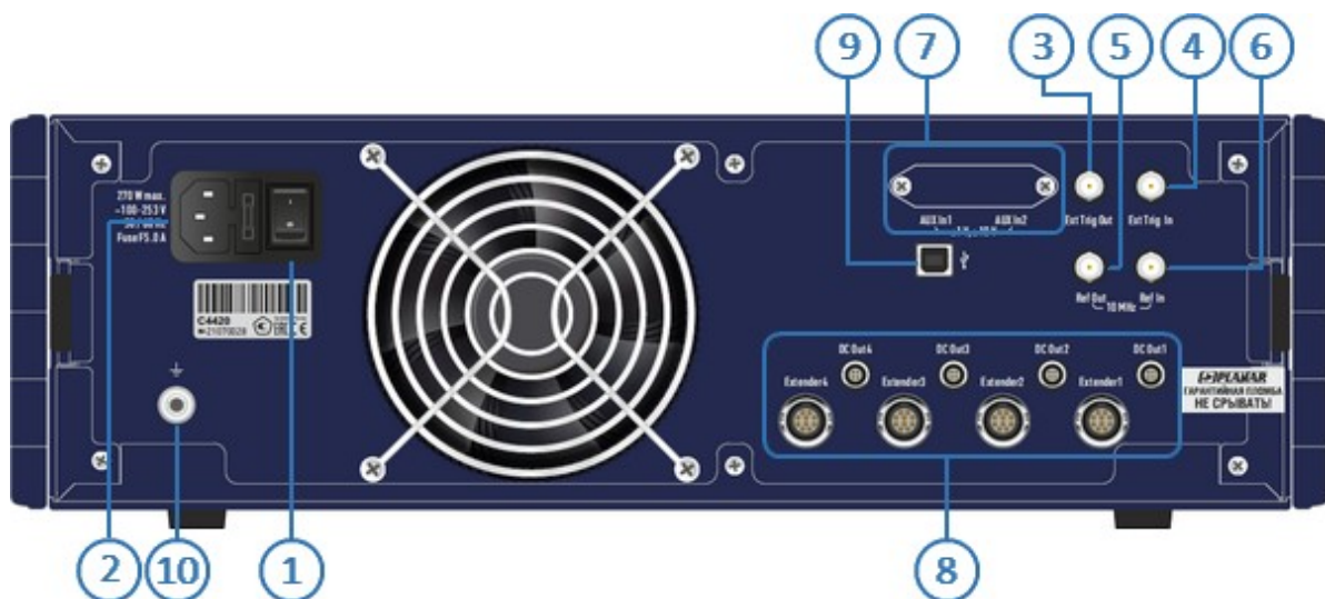
Рисунок – Задняя панель C4420
