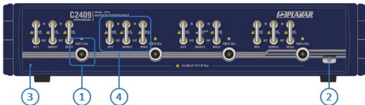
Рисунок – Передняя панель C2409
