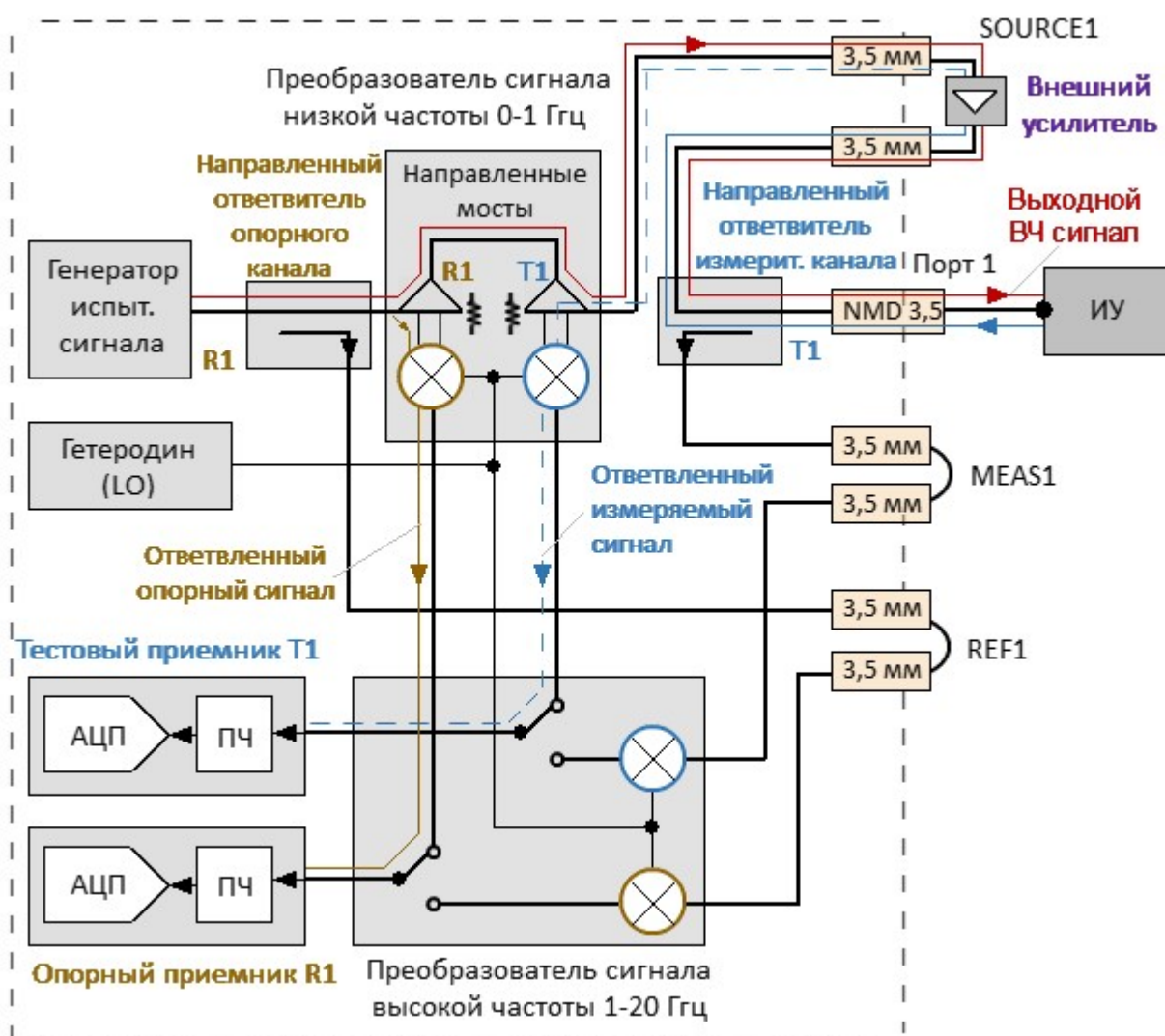
Рисунок – Анализатор C2420, распространение сигнала с внешним усилителем в тракте генератора (диапазон от 100 кГц до 1 ГГц)
