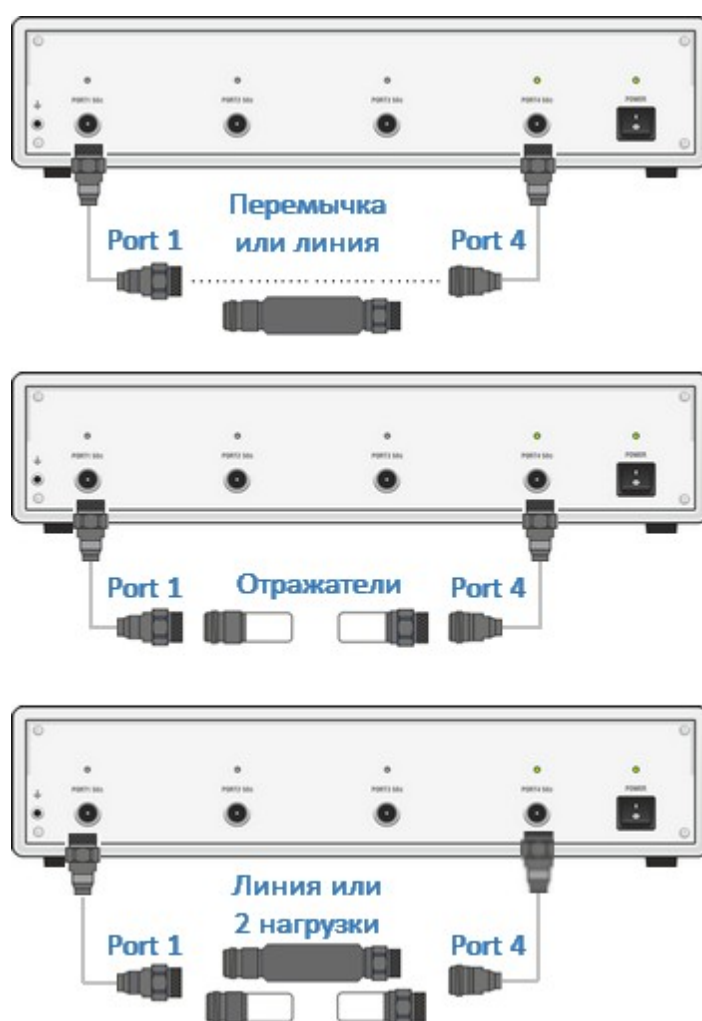
Рисунок – Калибровка TRL
