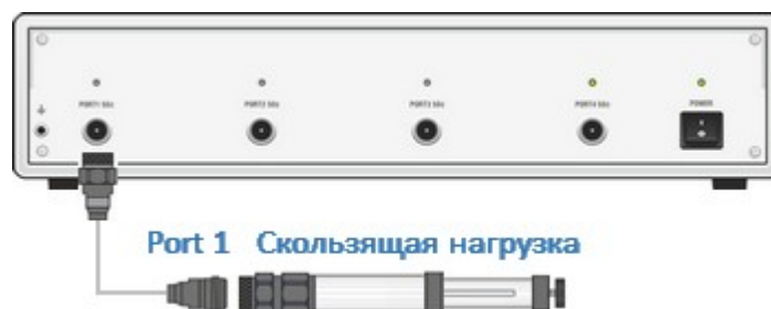
Рисунок – Калибровка скользящей нагрузкой
