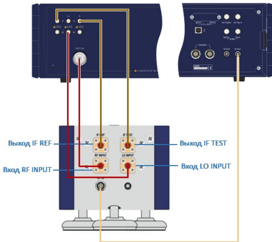
Рисунок – Схема подключения модуля FEV к анализатору
