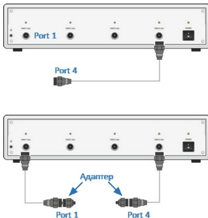
Рисунок – Примеры определения измерительных портов
