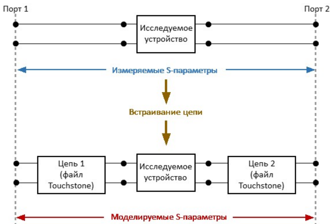
Рисунок – Встраивание цепи
