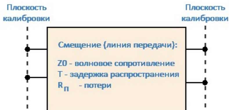
Рисунок – Модель двухпортовой меры
