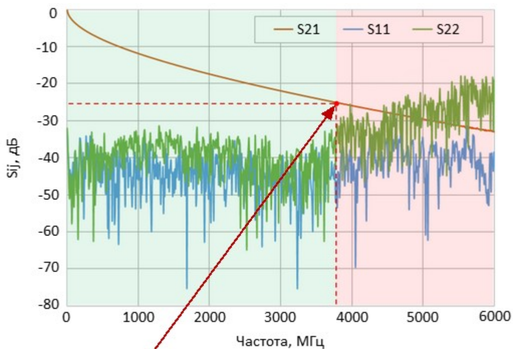
Рисунок – Коэффициенты передачи и отражения S_{11}^{ACMB} , S_{21}^{ACMB} , S_{22}^{ACMB}
