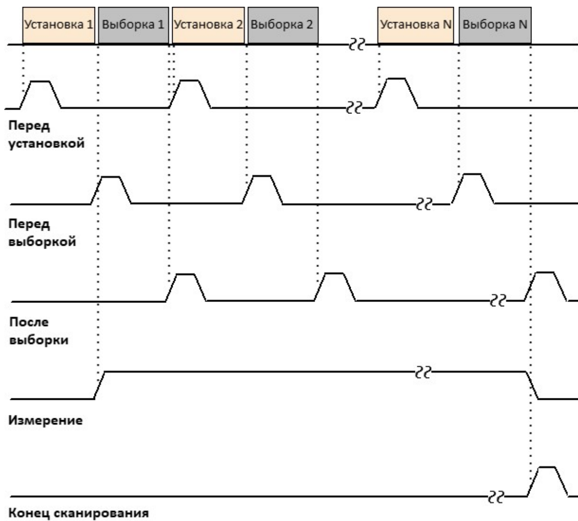
Рисунок — Выходной сигнала триггера (за исключением "готов к триггеру")
