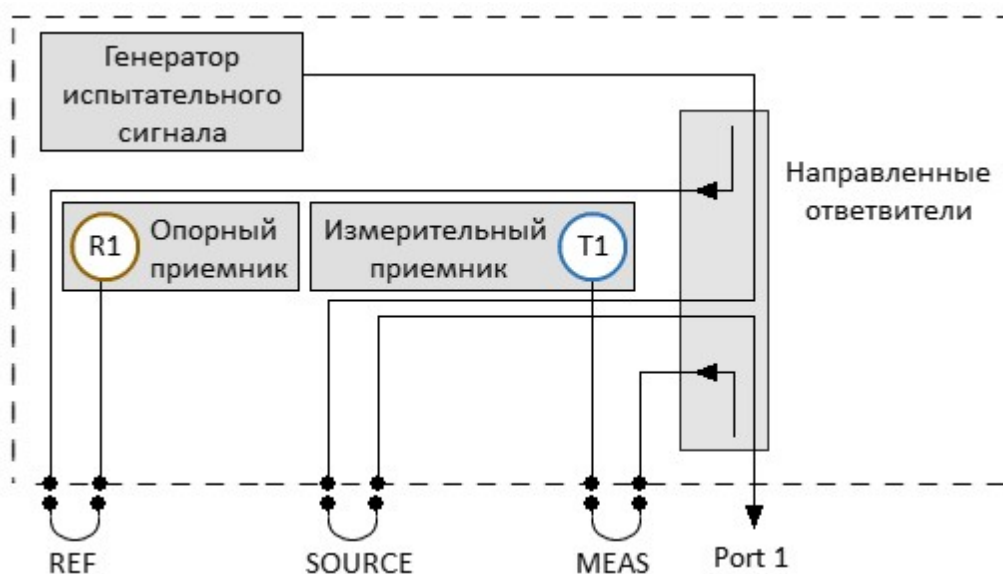
Рисунок – Схема прямого доступа к приемникам
