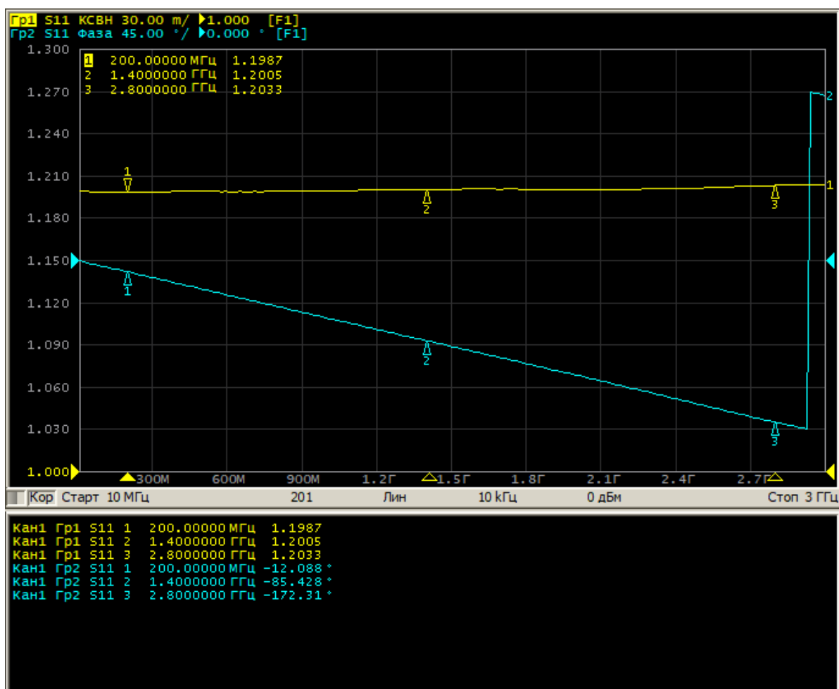
Рисунок – Пример измерения КСВН и фазы коэффициента отражения
