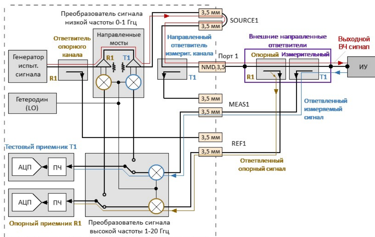
Рисунок – Анализатор C2420, распространение сигнала в режиме прямого доступа
