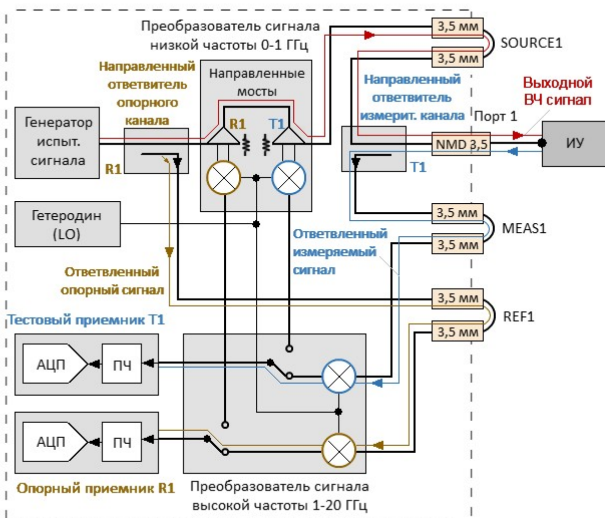
Рисунок – Анализатор C2420, распространение сигнала в общем режиме (диапазон от 1 до 20 ГГц)
