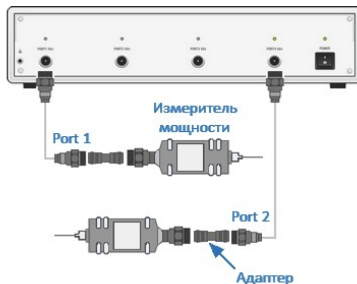
Рисунок – Калибровка мощности с помощью внешнего измерителя мощности
