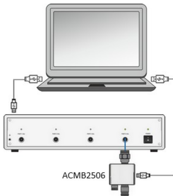
Рисунок – Схема подключения ACMB2506 для калибровки и настройки
