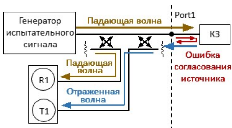
Рисунок – Ошибка согласования источника
