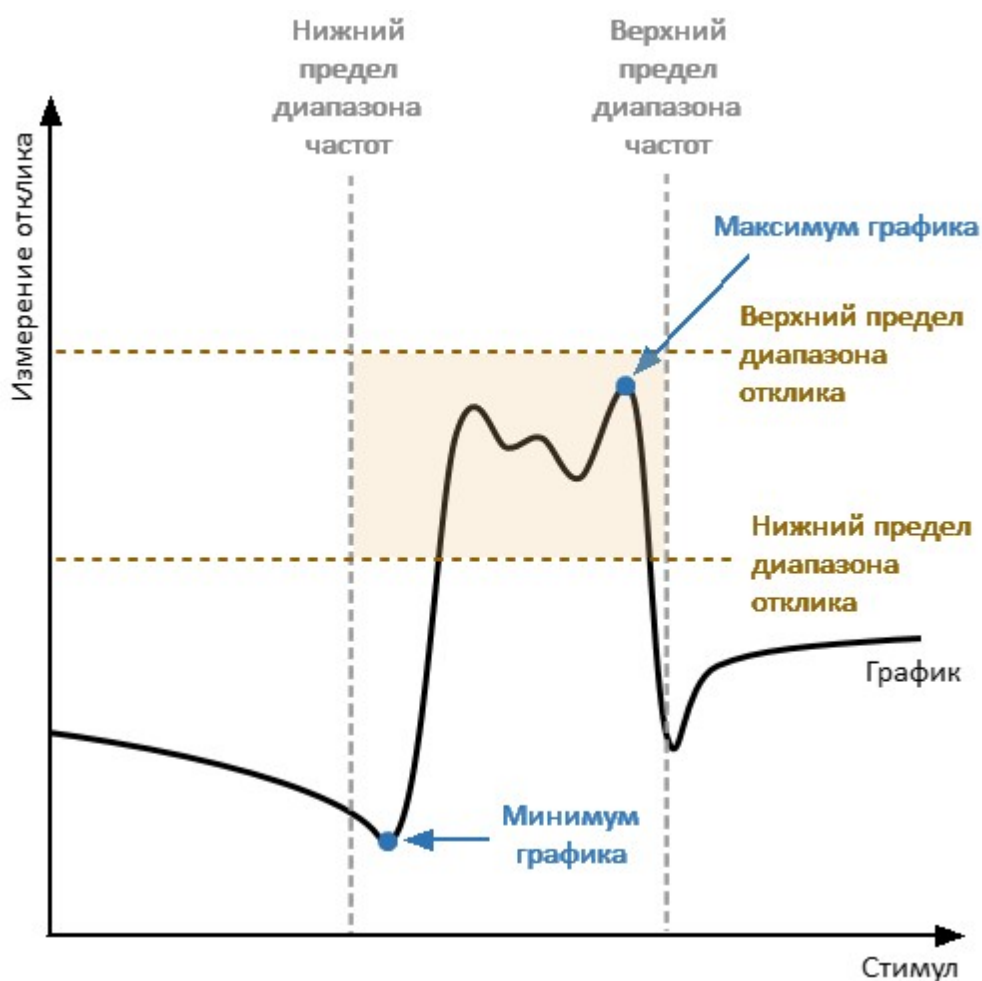
Рисунок – Тест пределов для пика
