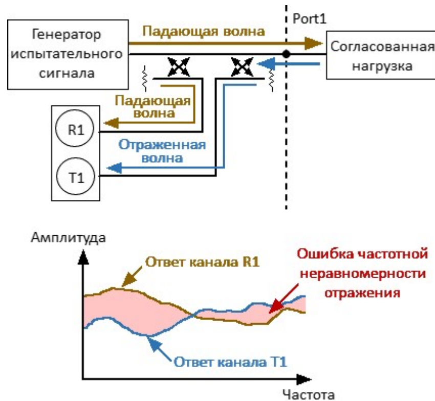
Рисунок – Ошибка частотной неравномерности отражения
