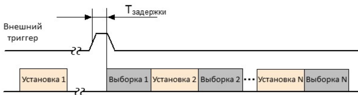
Рисунок — Задержка внешнего триггера
