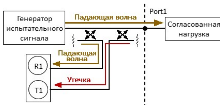
Рисунок – Ошибка направленности
